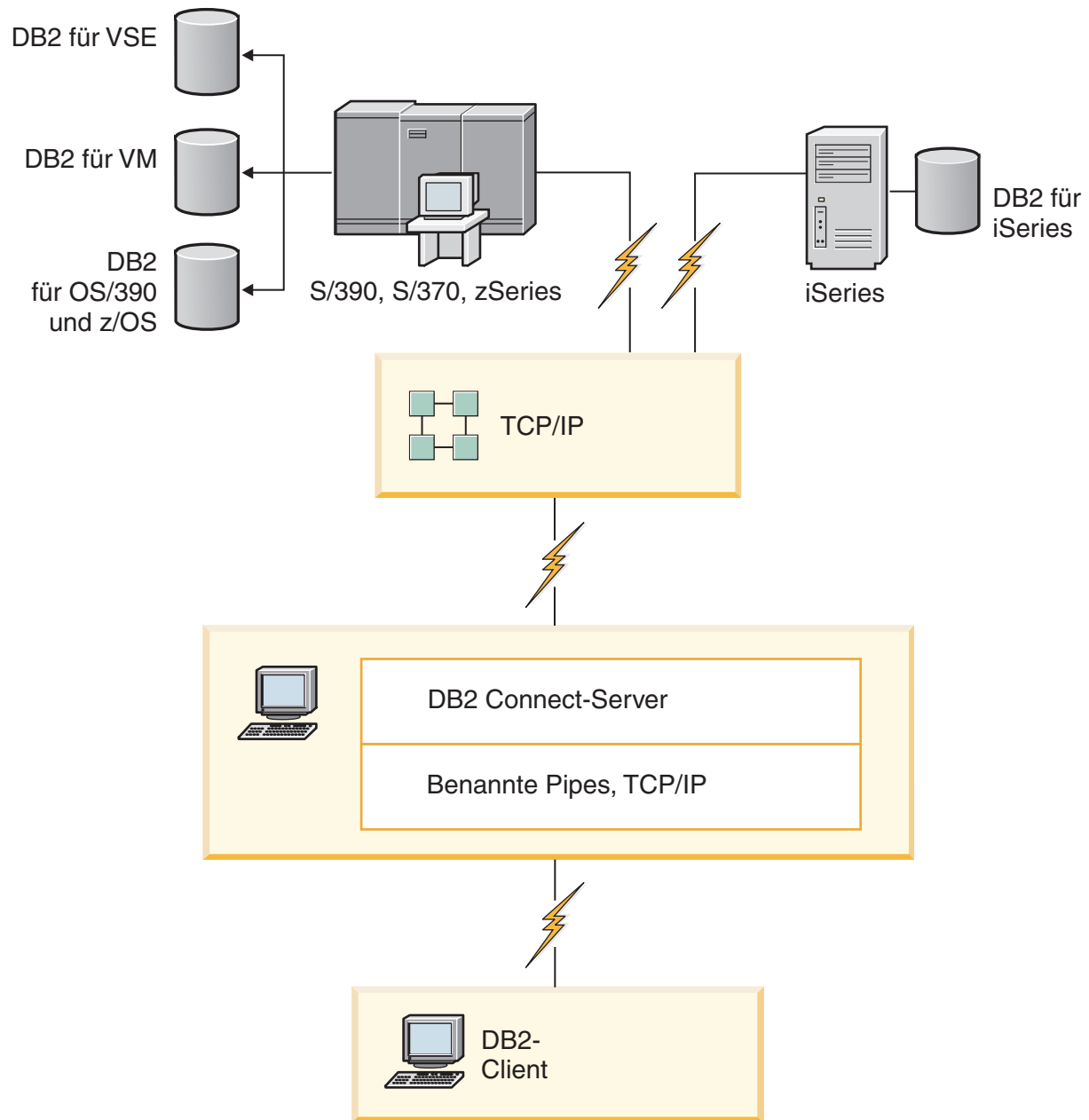
Abbildung 2. Herstellen einer Clientverbindung zu einem Host- oder System i-Datenserver mithilfe von DB2 Connect
