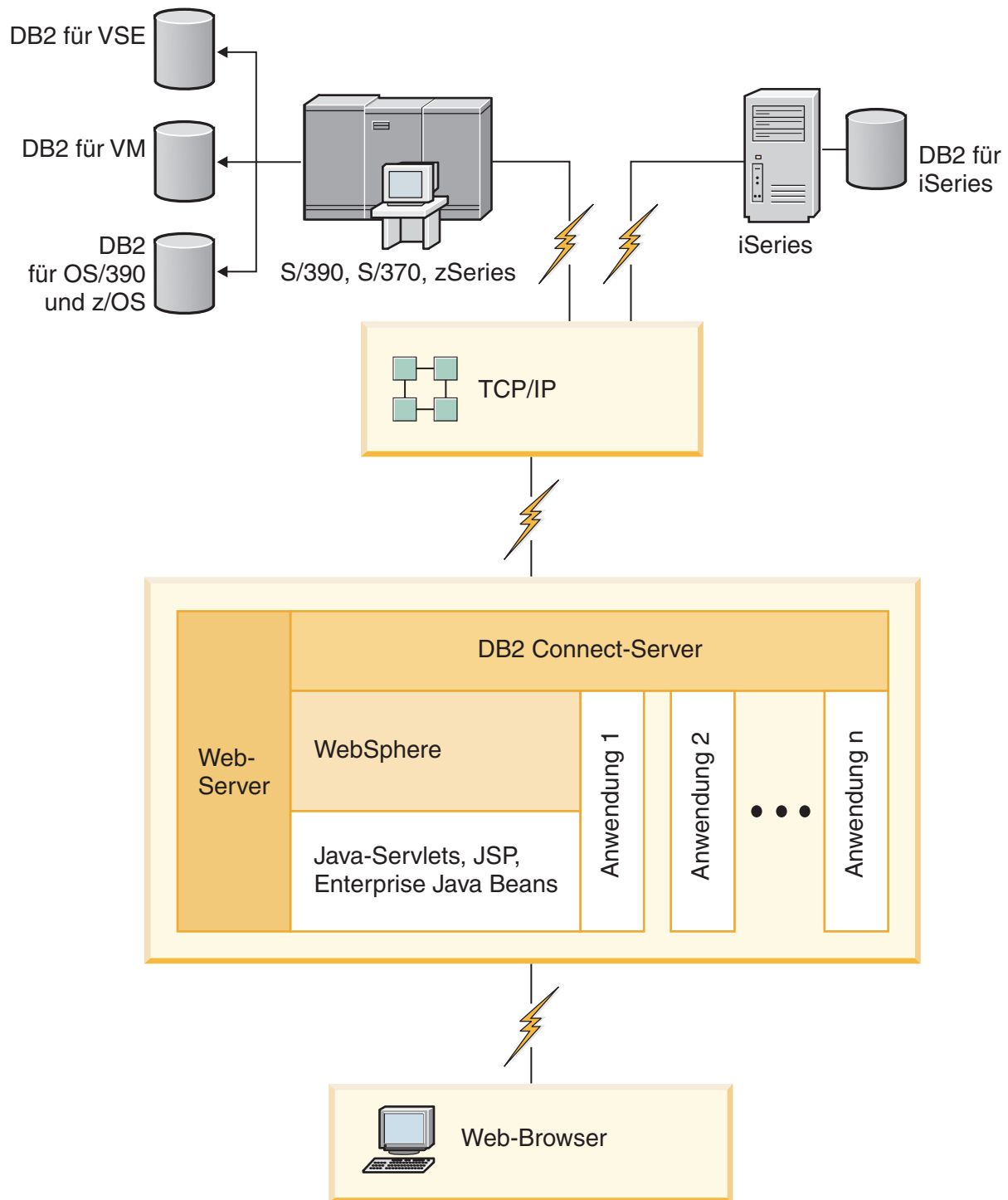
Abbildung 4. WebSphere- und Java-Serverfunktionalität in DB2 Connect
