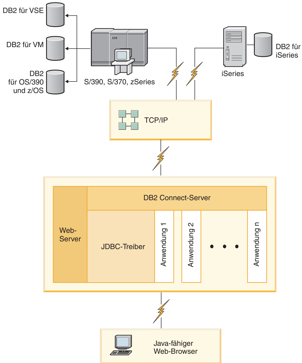
Abbildung 1. JDBC und DB2 Connect
