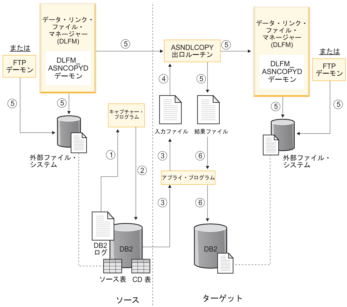
図6. DATALINK レプリケーション・プロセス
