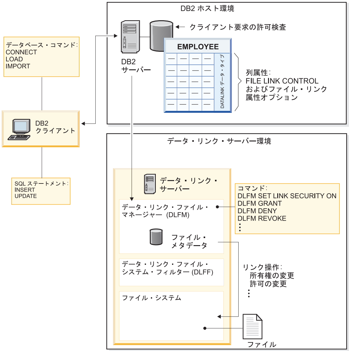
図3. ファイル・リンク処置および制御
