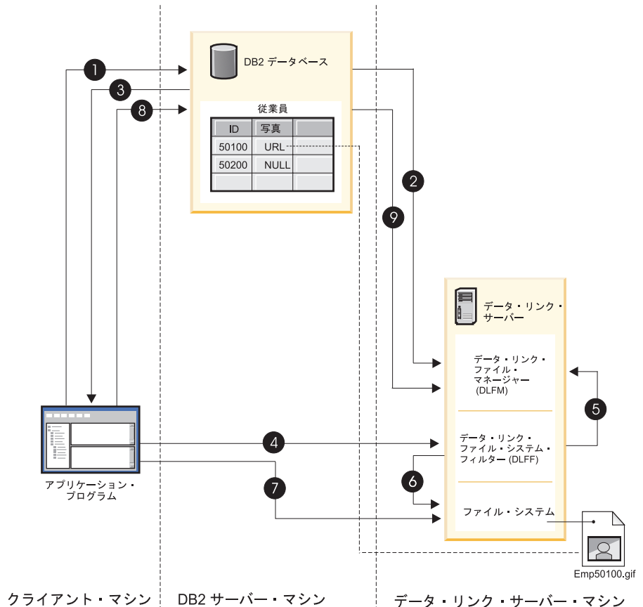
図 5. アプローチ 3 のアプリケーション・プログラムのフロー
