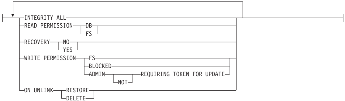
図 2. DATALINK 列定義の構文
