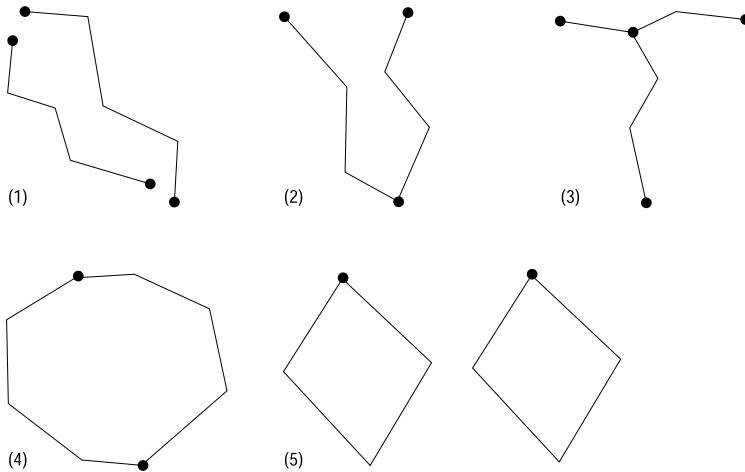
圖 12. 多線串。
