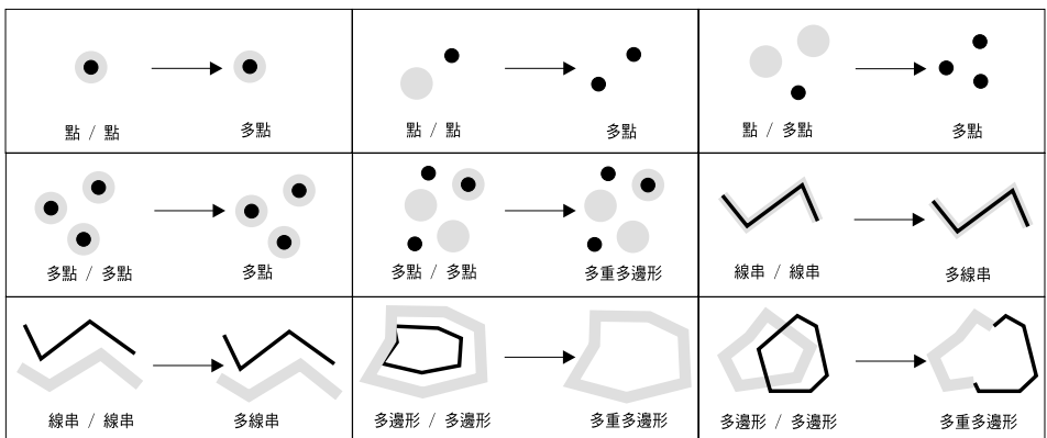
圖 23. ST_Union
