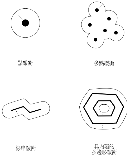
圖 24. ST_Buffer
