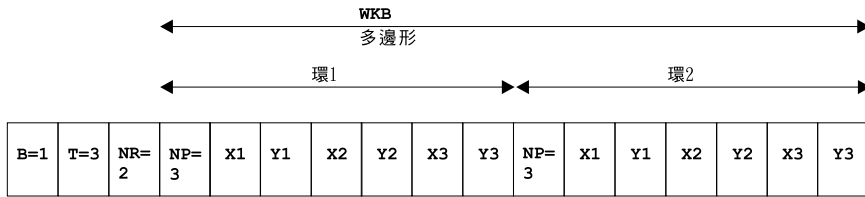
圖 39. 使用 NDR 格式的代表. 具有 2 線性 (NR=2) 的類型多邊形 (T=3) 的 (B=1), 每一個環有 3 點 (NP=3)。
