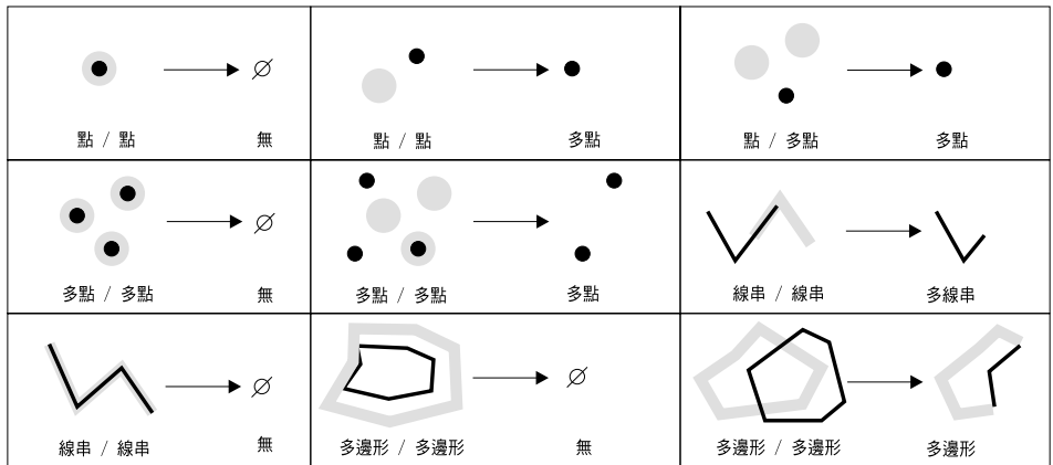
圖 22. ST_Difference
