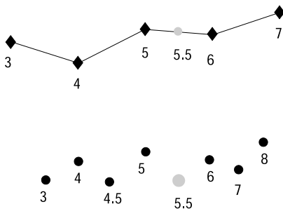
圖 25. LocateAlong
