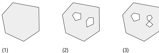
圖 11. 多邊形.
