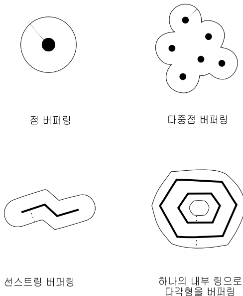
그림 24. ST_Buffer
