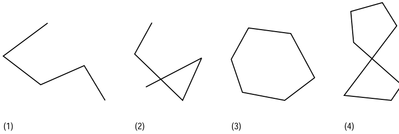
그림 10. 선스트링 오브젝트
