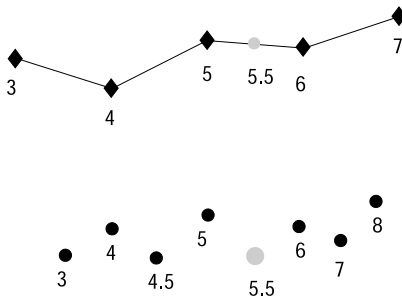
그림 25. LocateAlong
