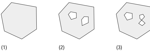
그림 11. 다각형.
