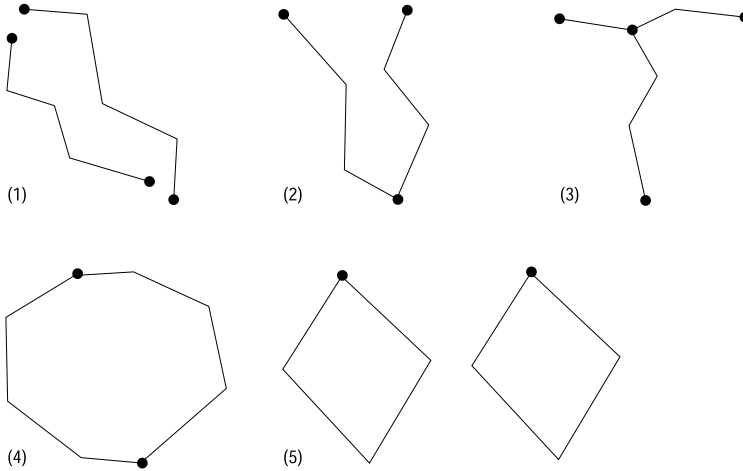
그림 12. 다중 선스트링.
