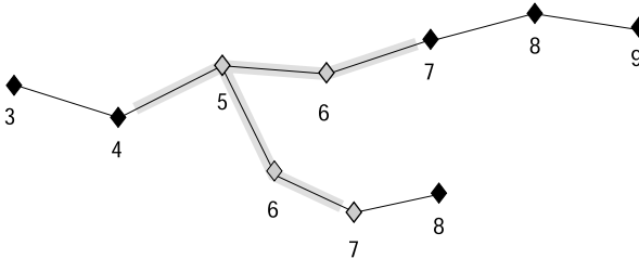
그림 26. LocateBetween
