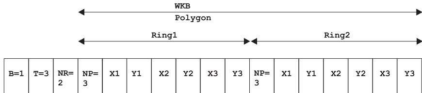
图 39. NDR 格式的表示. (B=1), 类型为多边形 (T=3), 具有 2 条直线 (NR=2), 每个环具有 3 个点 (NP=3).
