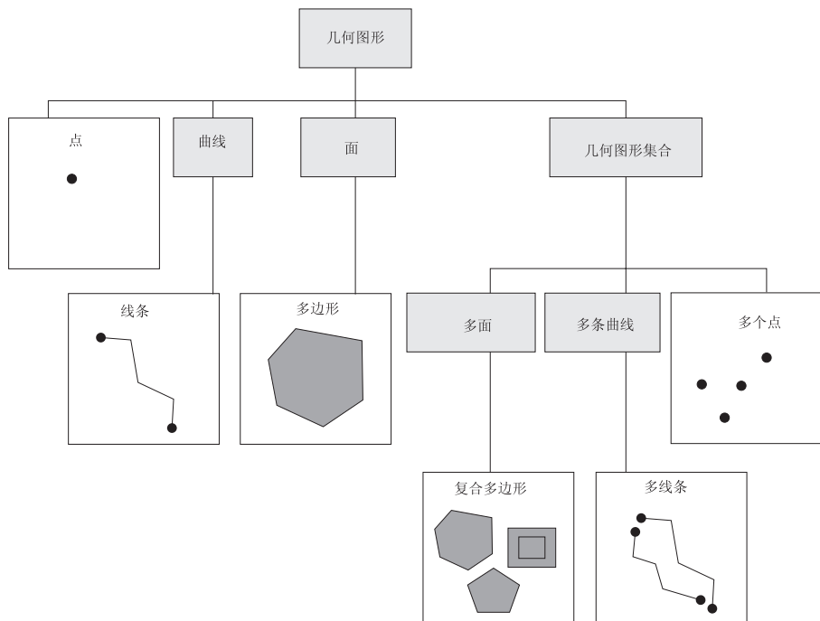
图9. Spatial Extender 支持的几何图形分层。可例示的几何图形可用直观符号表示。这些符号显示在这些几何图形名称下面。
