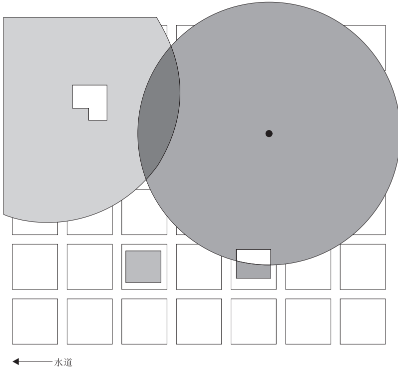
图 38. 使用 ST_SymmetricDiff 确定不包含敏感区域（居住建筑物）的有害废物区域 在图38中，有害废物地点和敏感区域的对称差异导致相交区域减小。
