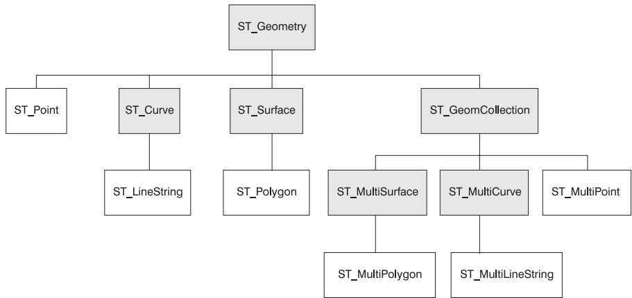
图 6. 空间数据类型的层次结构. 在白色框中命名的数据类型是可实例化的。在阴影框中命名的数据类型是不能实例化的。
