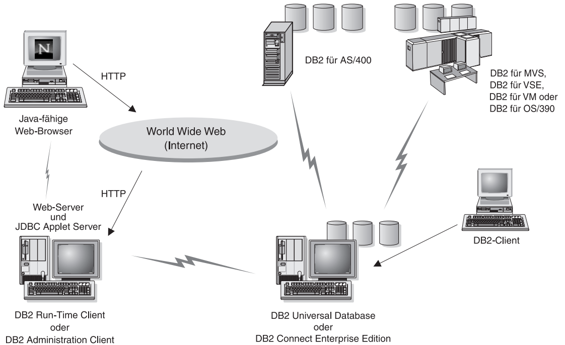
Abbildung 5. Zugreifen auf unter DB2 gespeicherte Daten mit Hilfe von JDBC
