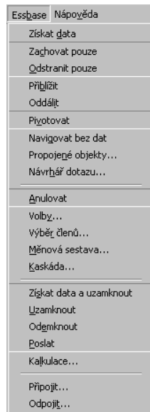
Obrázek 5. Nabídka Essbase
