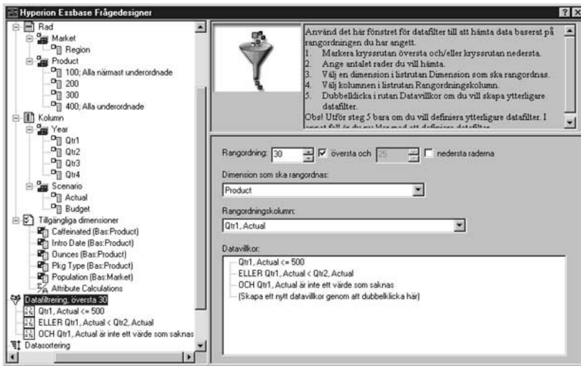
Figur 92. Datafiltrering
