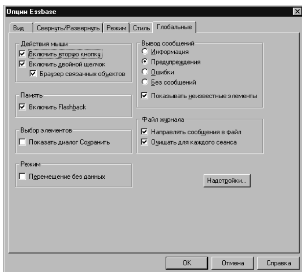
Рисунок 179. Исходные установки опций на странице Глобальные
