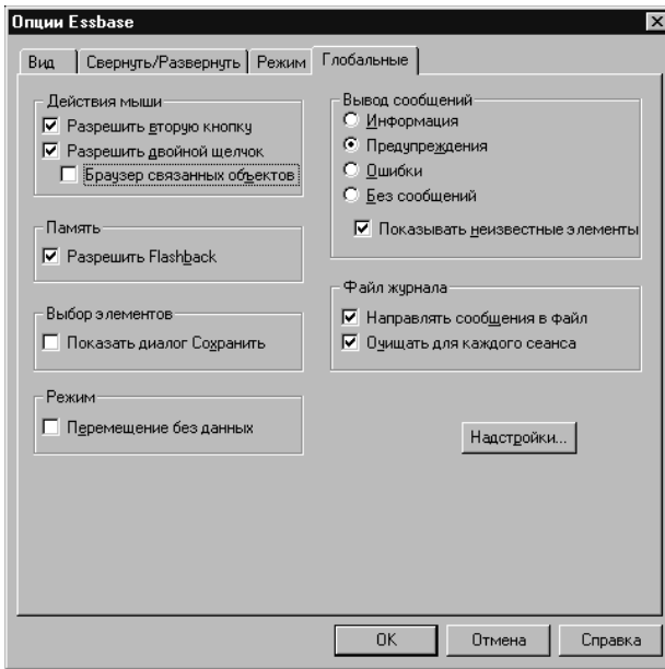
Рисунок 9. Диалоговое окно Опции Essbase — Вкладка Глобальные
