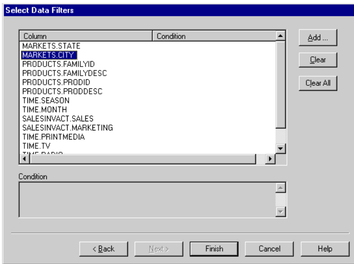
Рисунок 194. Диалоговое окно Выбор фильтров данных
