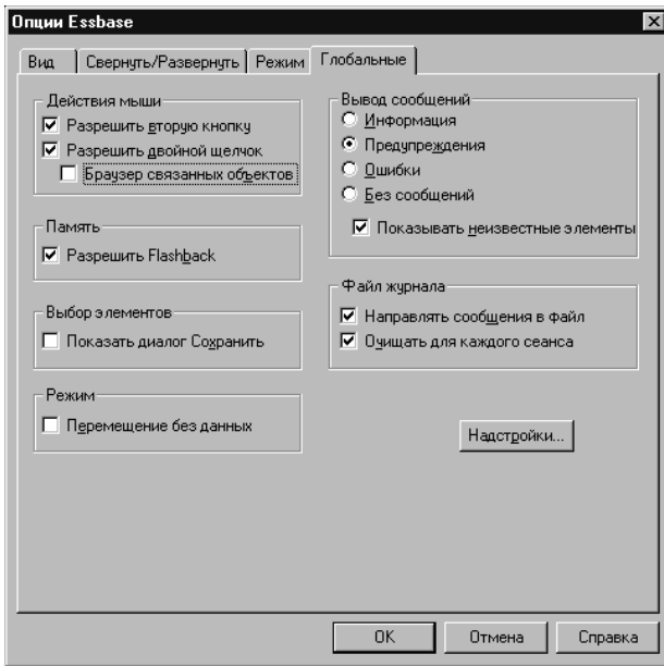
Рисунок 13. Исходные установки опций на странице Глобальные
