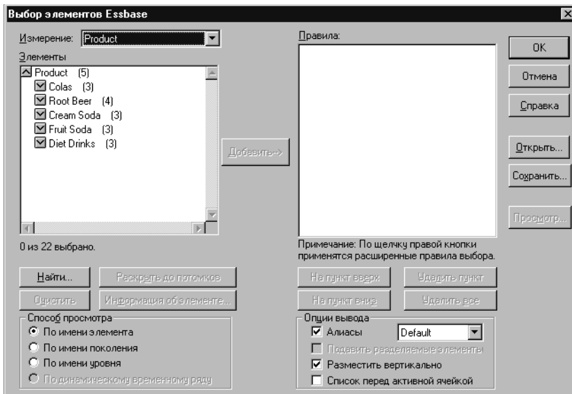
Рисунок 72. Диалоговое окно Выбор элементов Essbase
