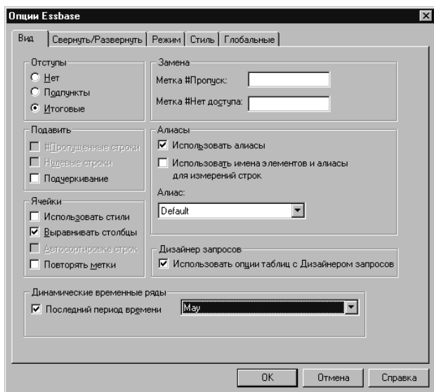
Рисунок 175. Исходные установки опций на странице Вид
