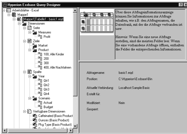
Abbildung 66. Hyperion Essbase Query Designer mit Abfrageinformationsanzeige
