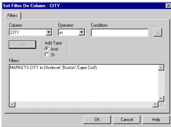
Abbildung 197. Definieren eines Filters für eine Spalte
