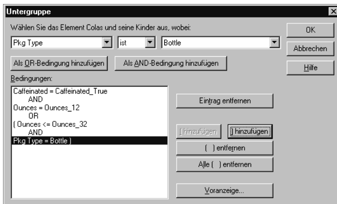
Abbildung 76. Dialogfenster "Untergruppe" (nach dem Hinzufügen von Bedingungen)
