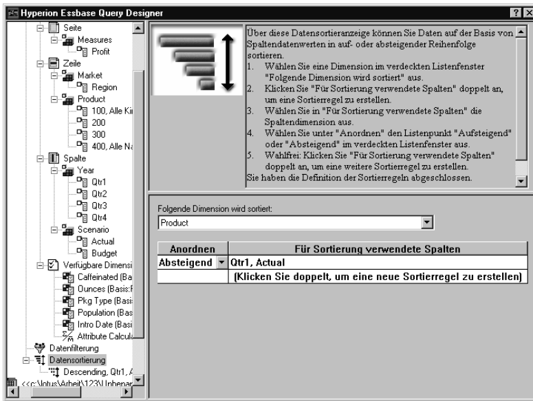
Abbildung 95. Festlegen der Datensortierreihenfolge
