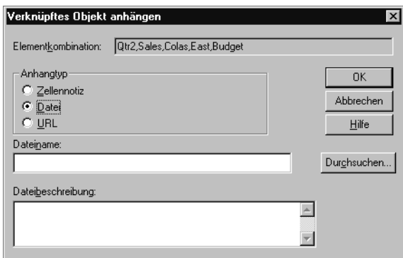
Abbildung 143. Verknüpfen einer Datei mit einer Datenzelle
