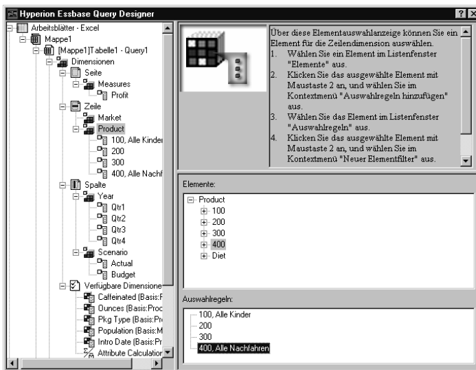
Abbildung 61. Auswählen von Elementen von Product
