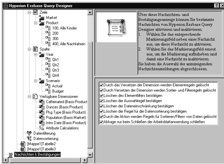
Abbildung 68. Nachrichten- und Bestätigungsanzeige
