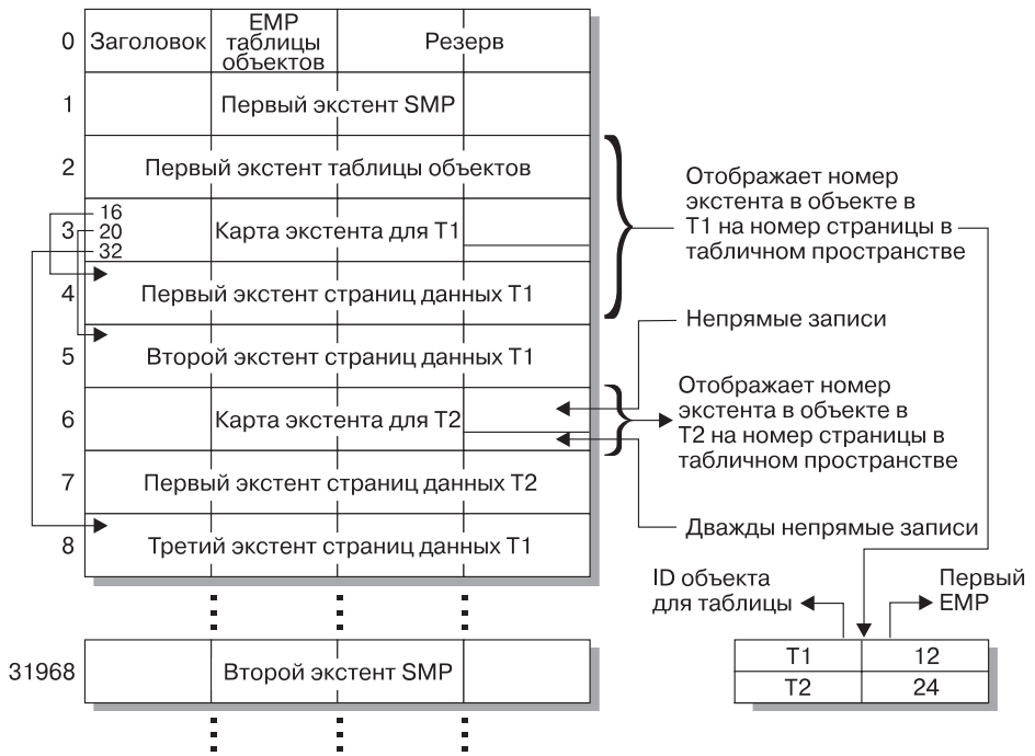
Рисунок 3. Табличные пространства DMS
