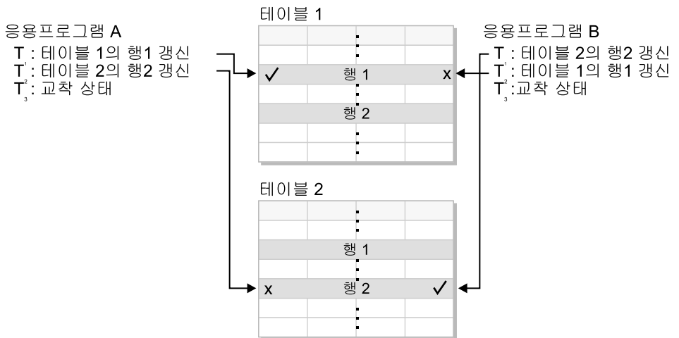
그림 2. 교착 상태 검출기
