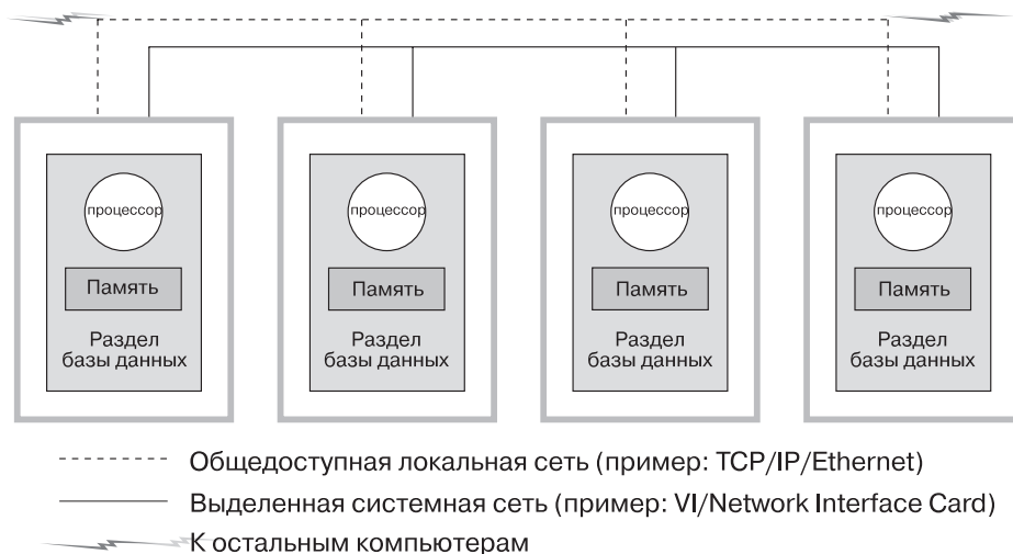
Рисунок 26. Объединение выделенной системной сети с общедоступной локальной сетью
