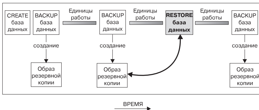
Рисунок 9. Восстановление базы данных с использованием образа резервной копии
