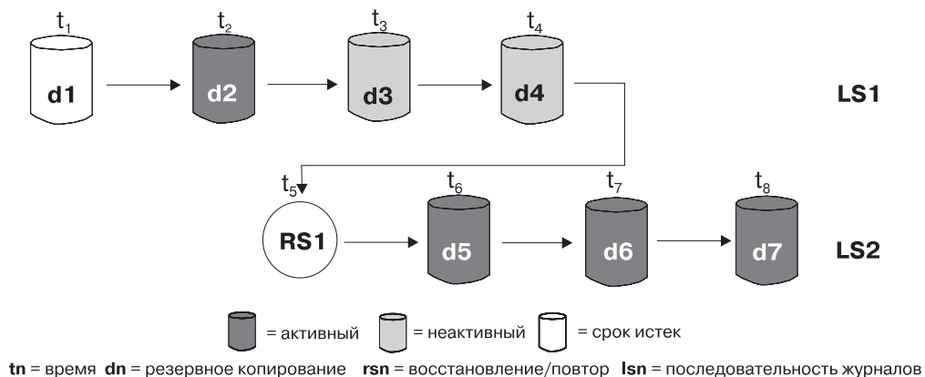
Рисунок 19. Резервные копии базы данных - активные, неактивные и с истекшим сроком
