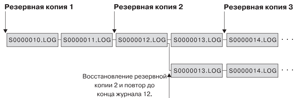
Рисунок 13. Повторное использование имен файлов журнала
