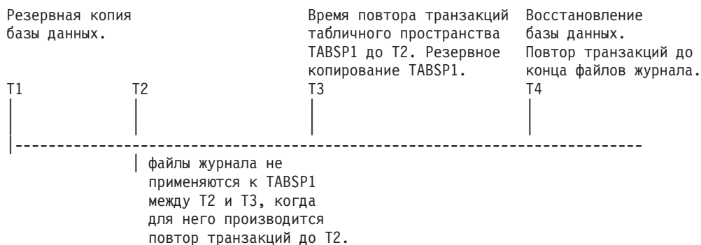
Рисунок 11. Требования к резервной копии табличного пространства
