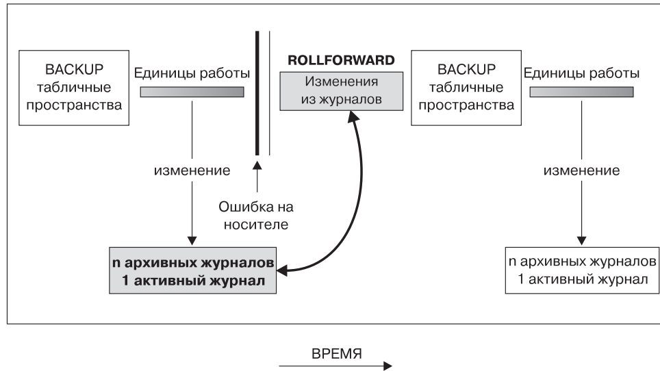
Рисунок 12. Восстановление с повтором транзакций табличного пространства
