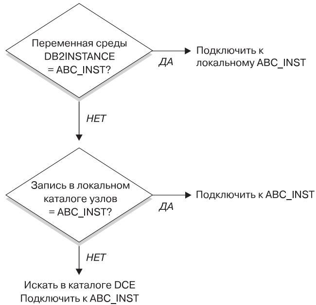
Рисунок 23. Как используются каталоги при подключении к базе данных
