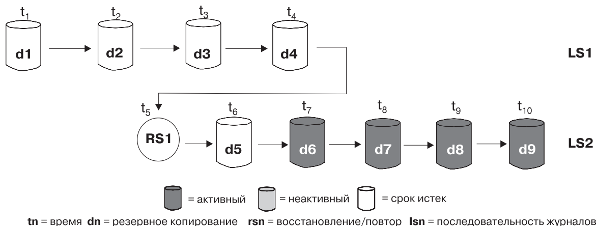
Рисунок 20. Последовательность файлов журнала с истекшим сроком годности
