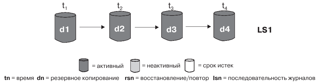
Рисунок 17. Активные резервные копии базы данных
