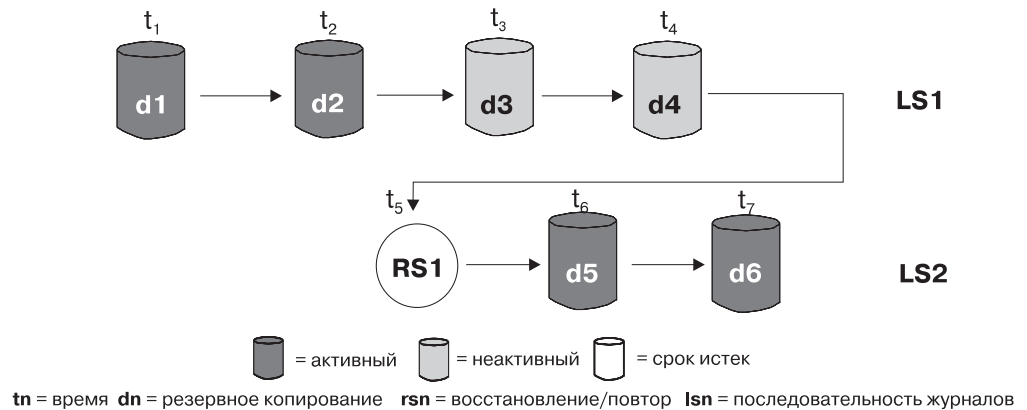
Рисунок 18. Неактивные резервные копии базы данных
