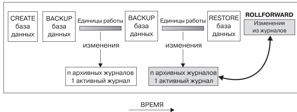
Рисунок 10. Восстановление с повтором транзакций
