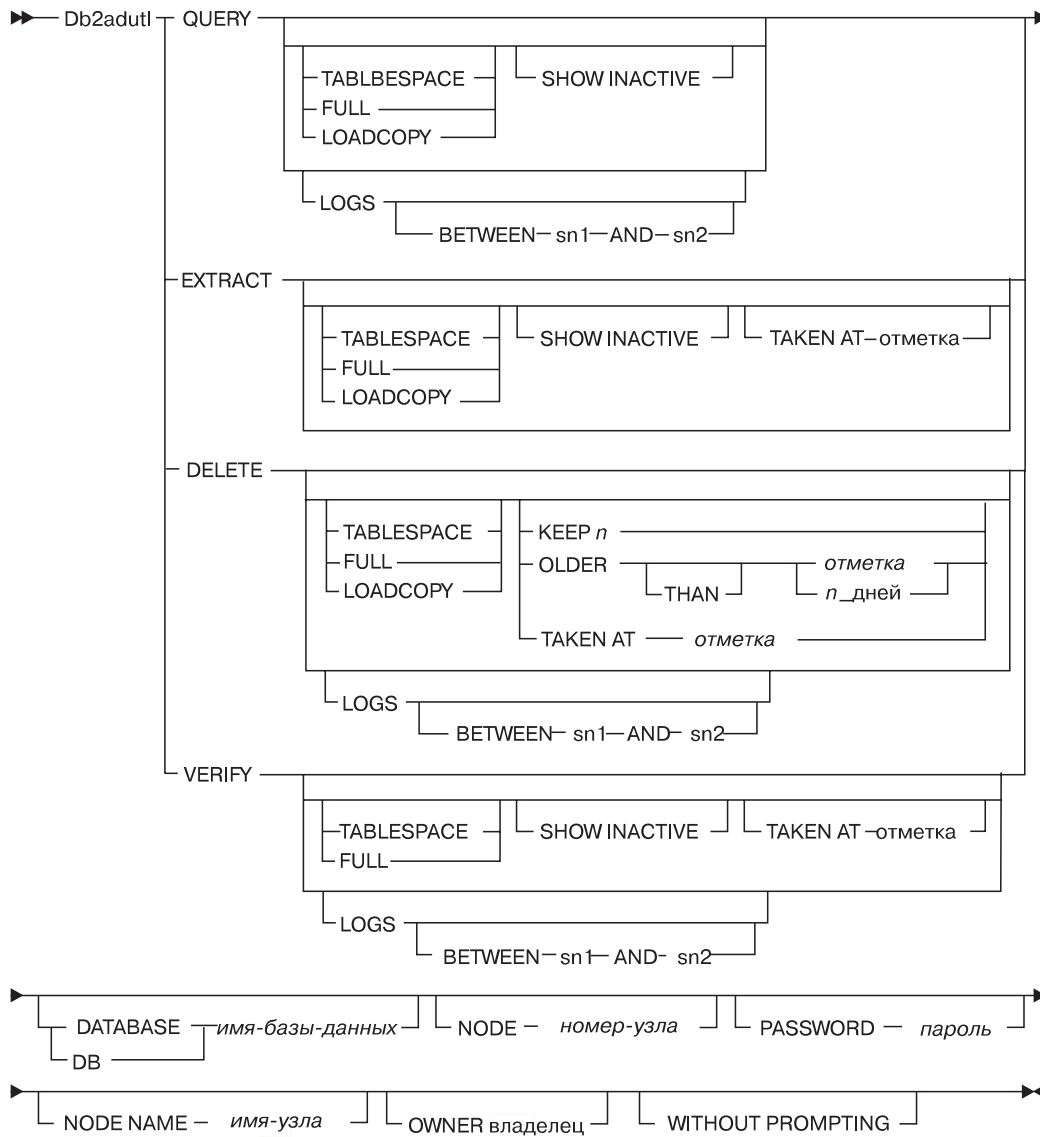
Рисунок 21. Синтаксис для db2adutl
