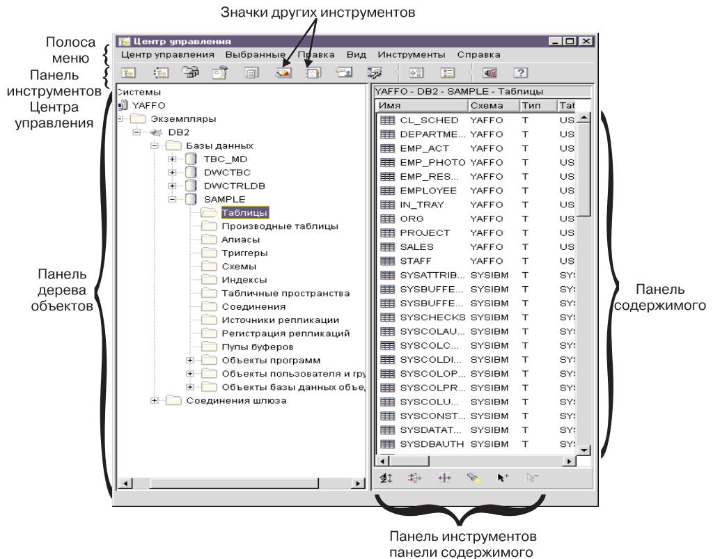
Рисунок 1. Возможности Центра управления
