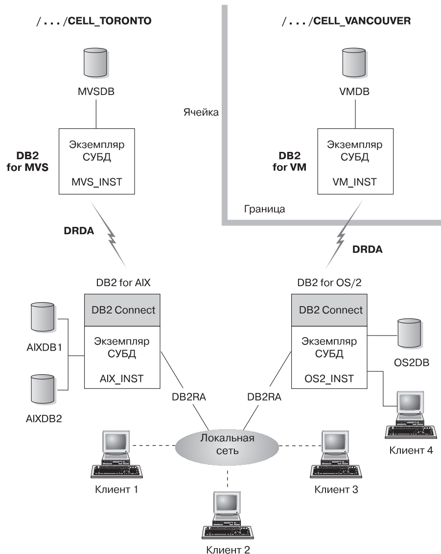
Рисунок 22. Конфигурация сетевой базы данных
