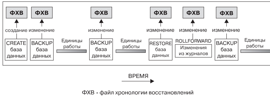
Рисунок 14. Создание и обновление файла хронологии восстановления
