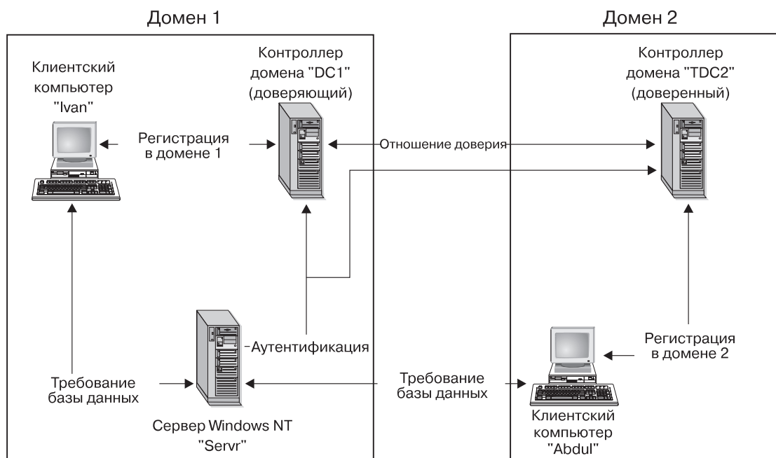
Рисунок 25. Аутентификация при помощи доменов Windows NT
