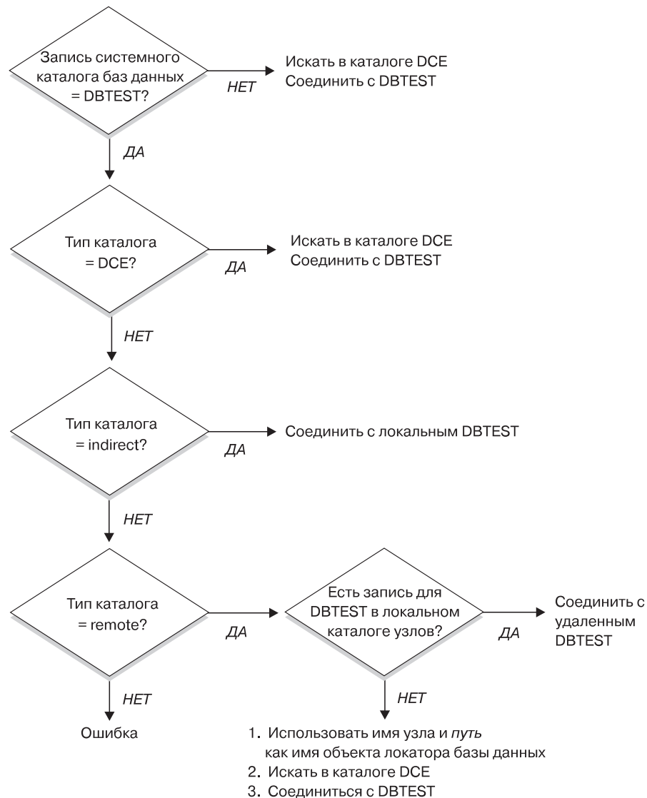
Рисунок 24. Как используются каталоги при соединении с базой данных
