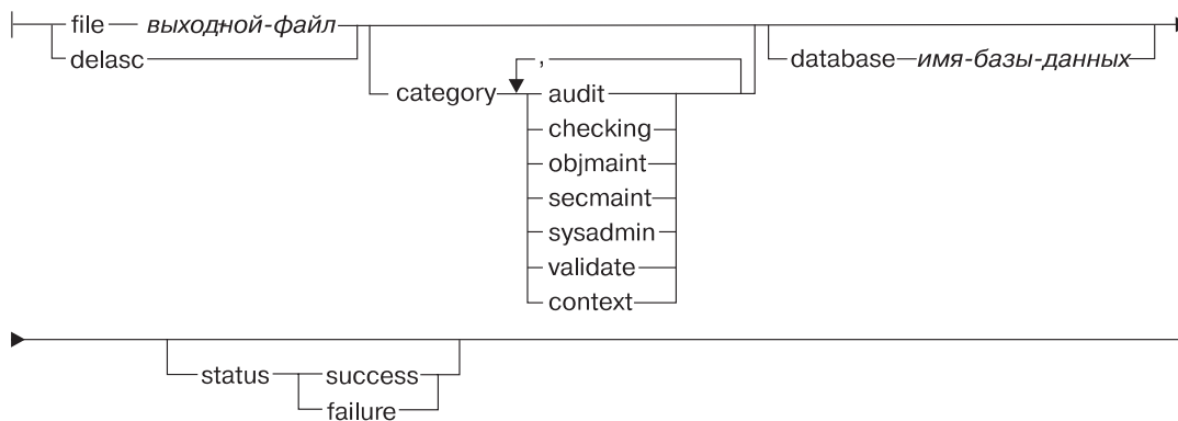
Рисунок 7. Синтаксис DB2AUDIT
