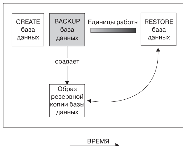
Рисунок 8. Создание образа базы данных
