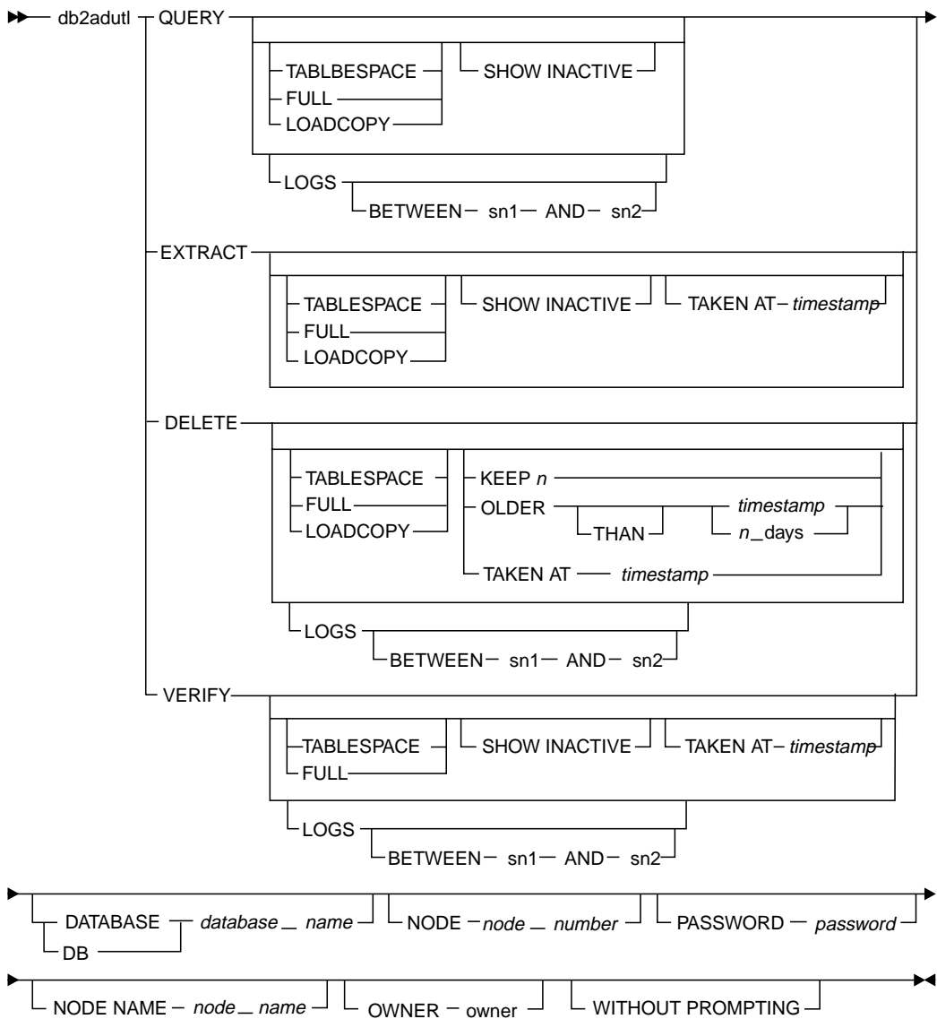
図 21. db2adutl の構文
