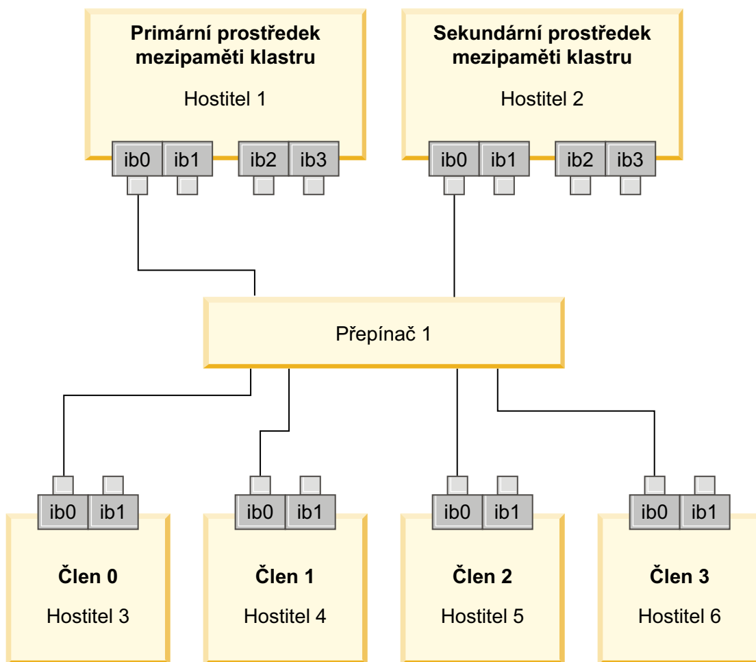
Obrázek 22. Dva moduly CF a čtyři členové se připojují k jednomu přepínači.
