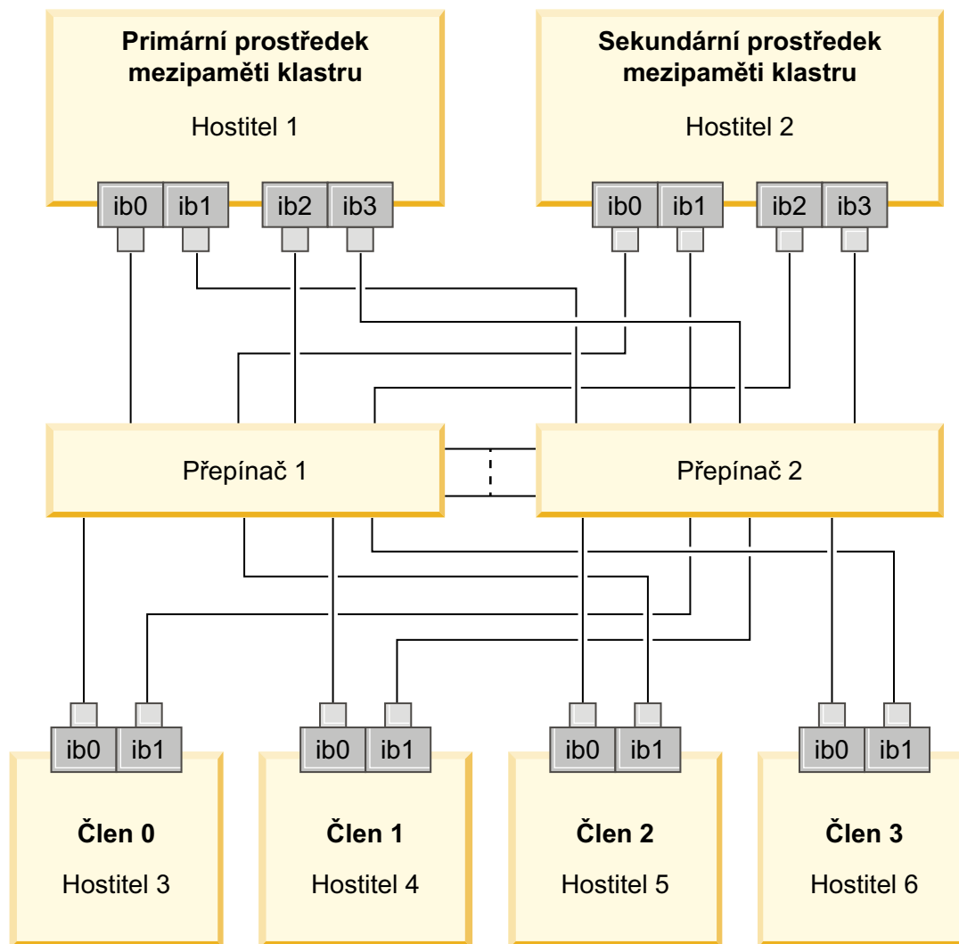
Obrázek 21. Dva moduly CF a čtyři členové se připojují ke dvěma přepínačům.
