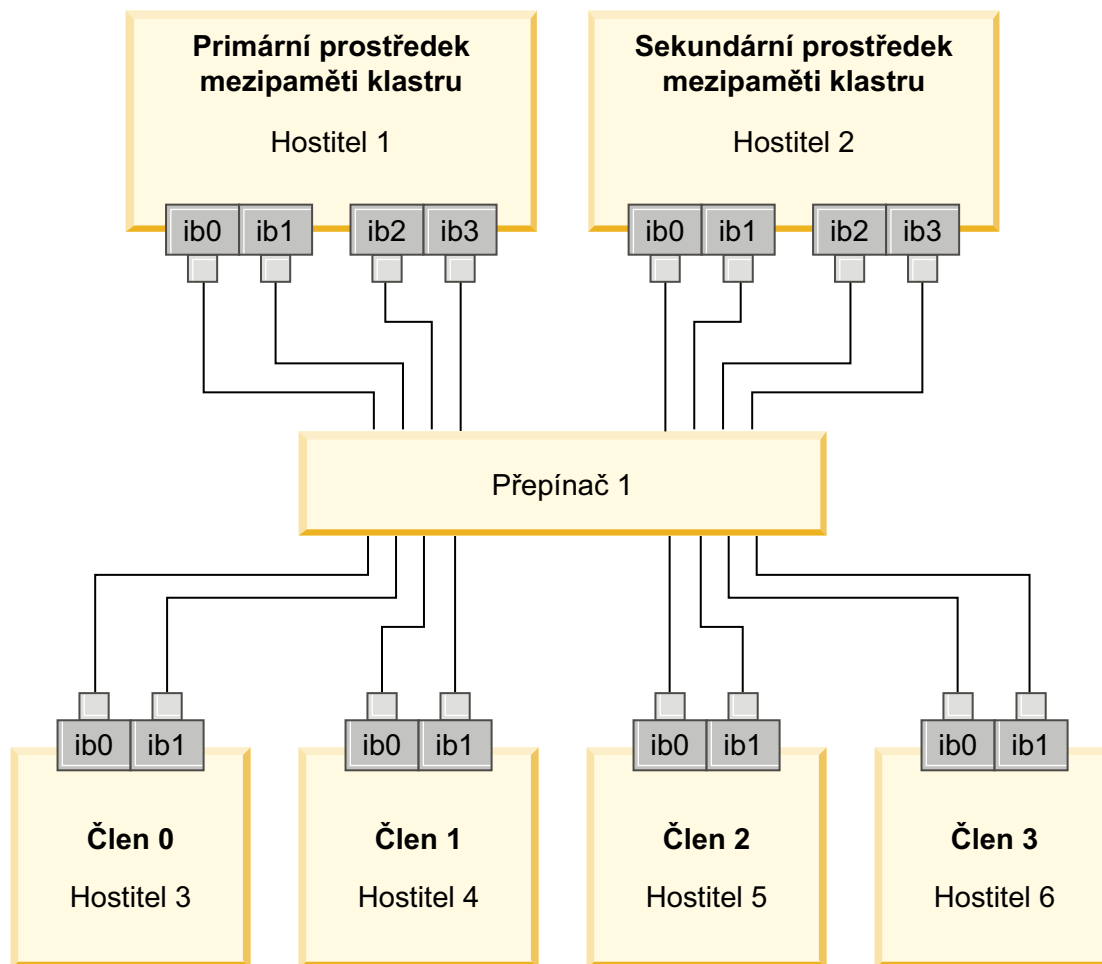
Obrázek 20. Dva moduly CF a čtyři členové se připojují k jednomu přepínači.
