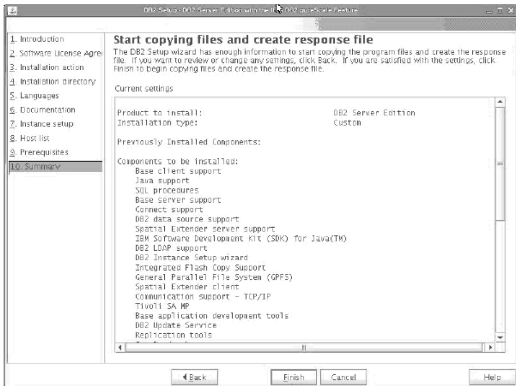
Obrázek 46. Panel Souhrn
