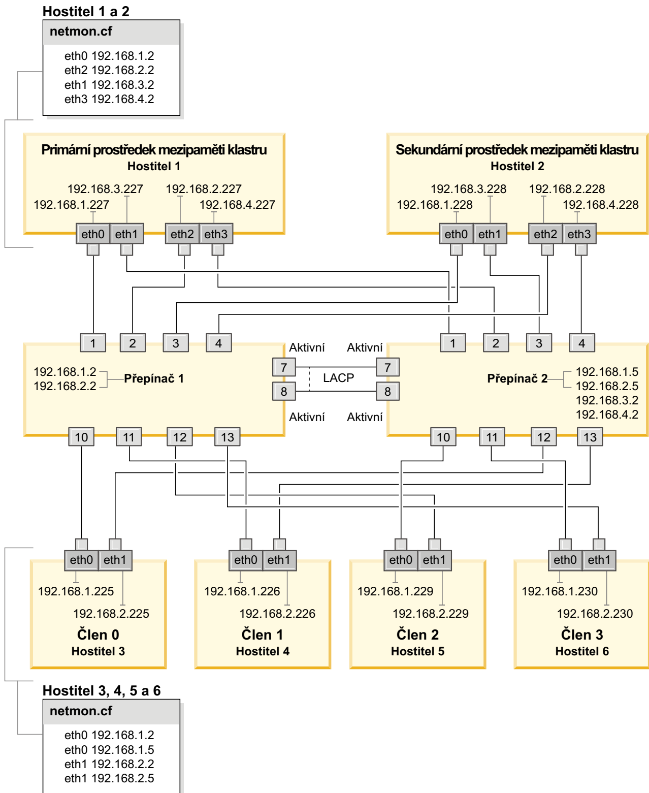
Obrázek 25. Dva moduly CF a čtyři členové se připojují ke dvěma přepínačům.
