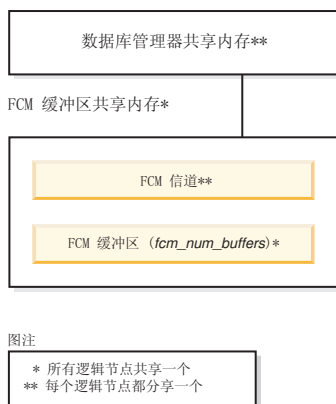
图 18. 使用多逻辑分区时的 FCM 缓冲池
