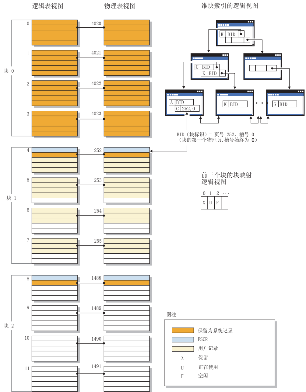
图 10. MDC 表和 ITC 表的逻辑表、记录和索引结构
