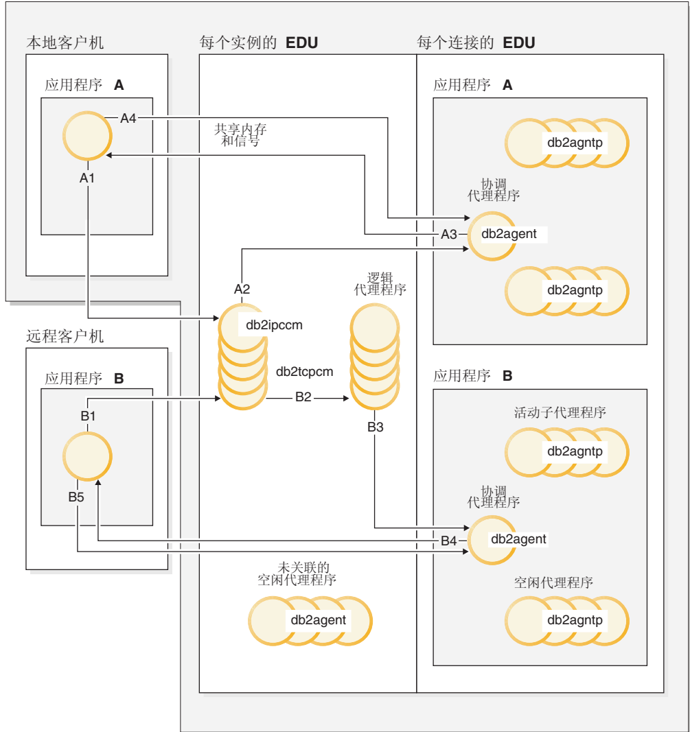
图 5. 客户机/服务器处理模型概述
