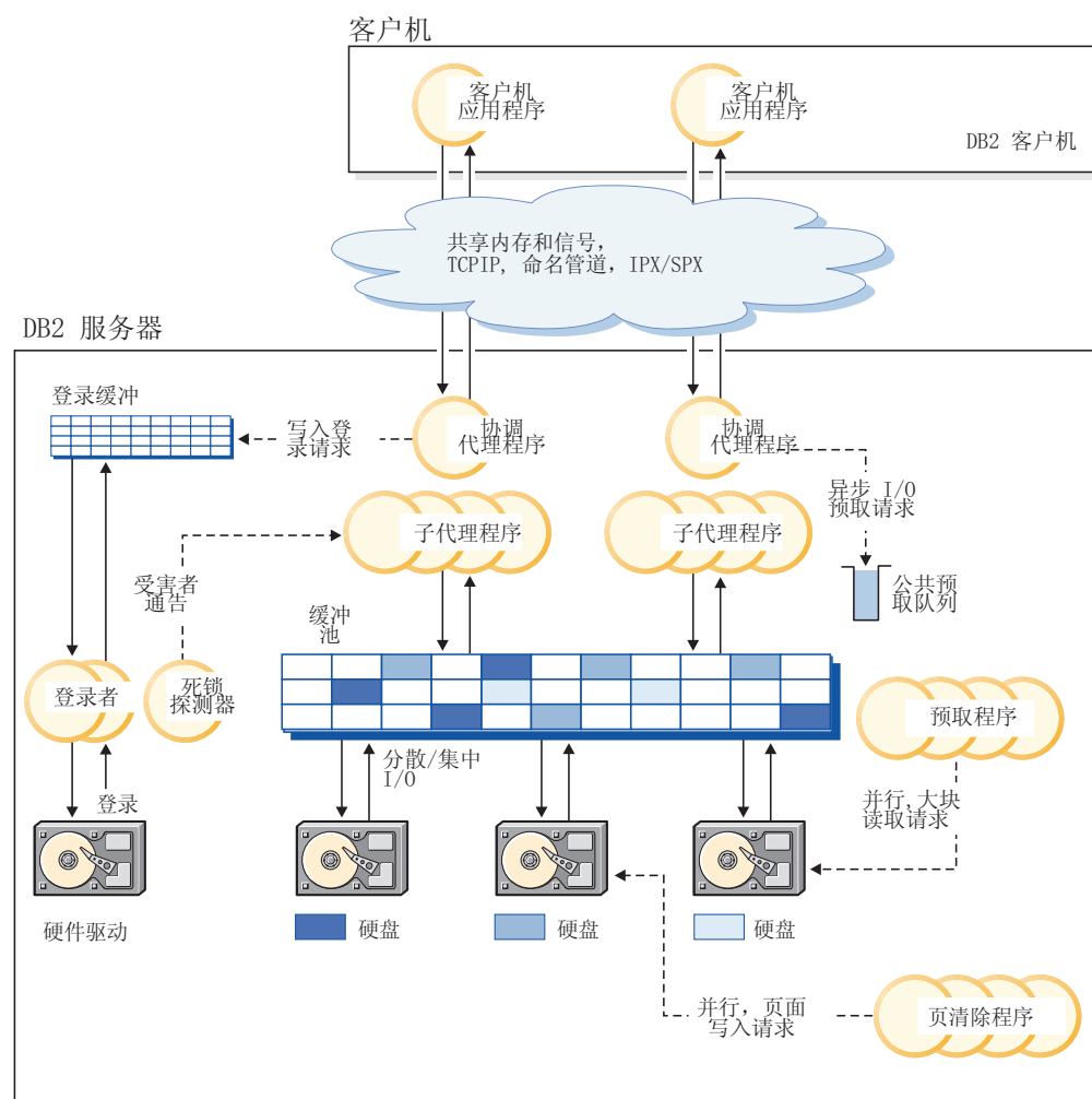
图 3. 客户机连接和数据库服务器组件
