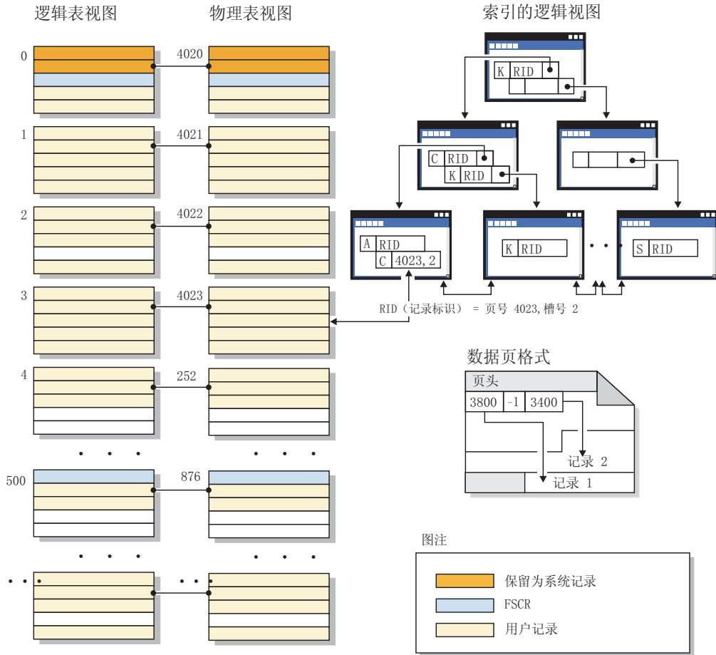
图 8. 标准表的逻辑表、记录和索引结构
