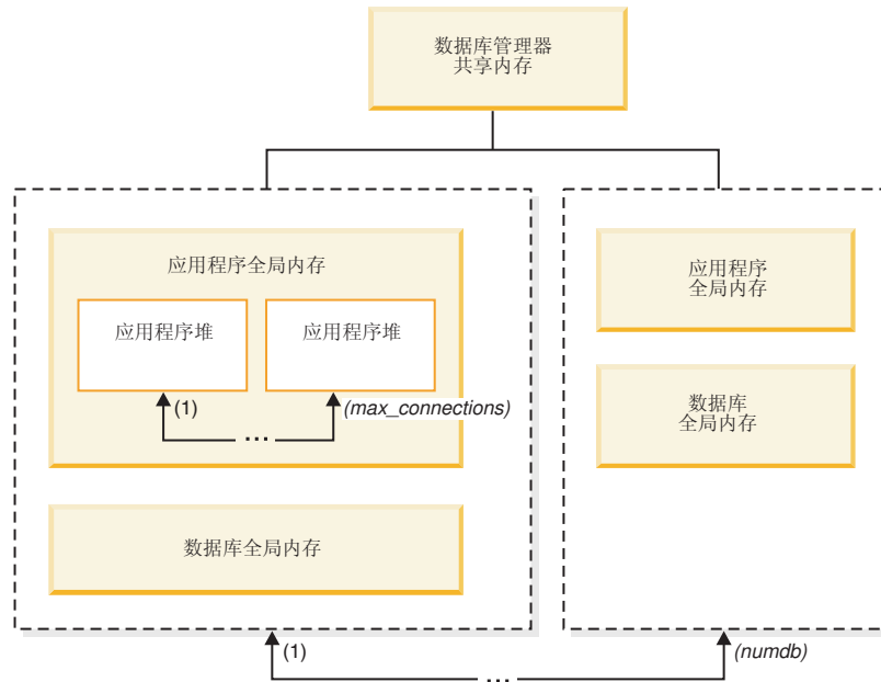
图 16. 数据库管理器分配的内存的类型
