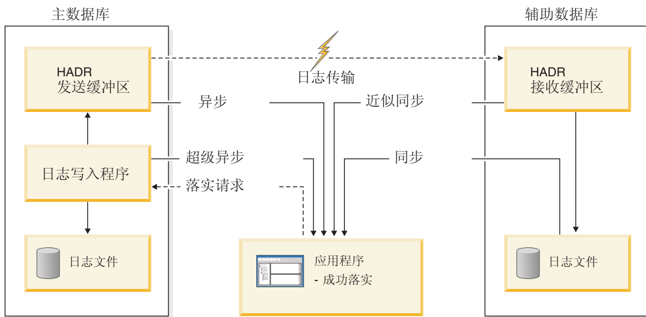
图 52. 高可用性和灾难恢复 (HADR) 的同步方式
