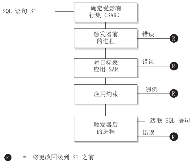
图 49. 处理包含相关触发器和约束的语句
