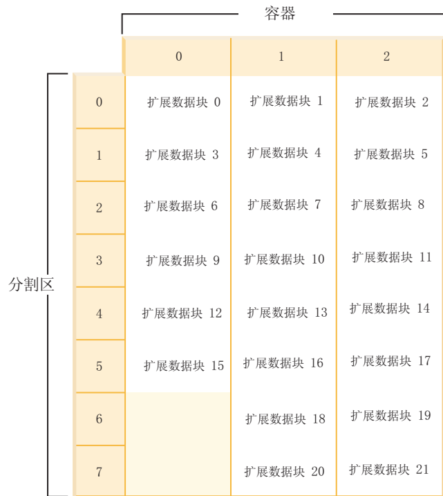
图 21. 带有三个容器和 22 个扩展数据块的表空间
