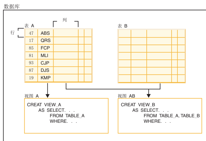
图 50. 表与视图之间的关系
