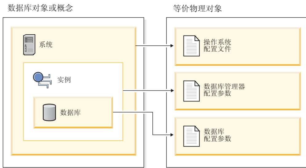
图 51. 数据库对象与配置文件之间的关系
