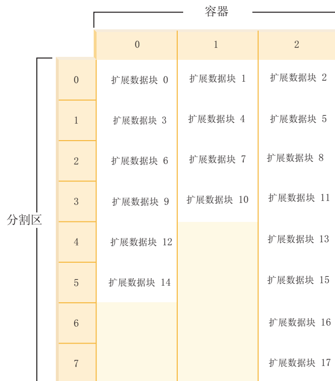
图 19. 带有三个容器和 18 个扩展数据块的表空间
