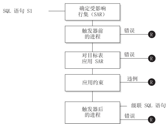
图 40. 处理包含相关触发器和约束的语句
