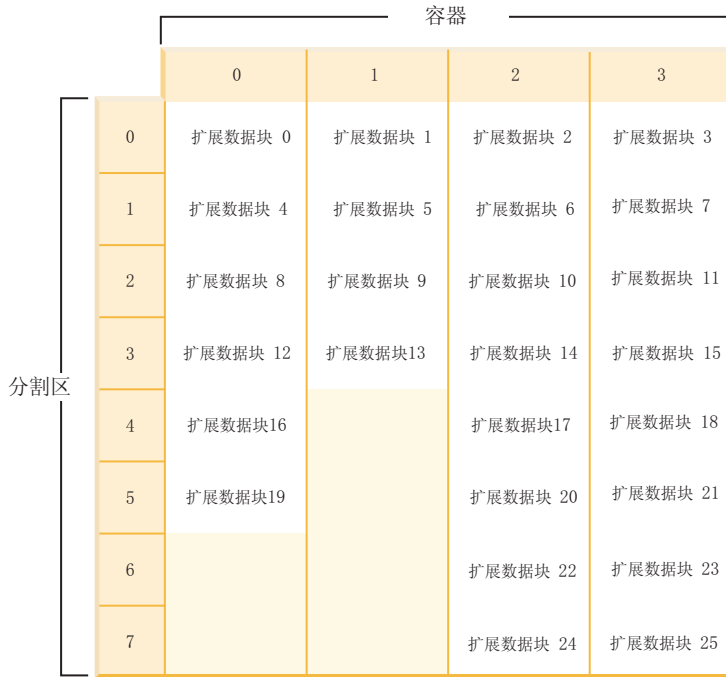
图 20. 带有四个容器和 26 个扩展数据块的表空间
