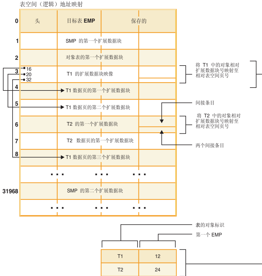
图 10. DMS 表空间
