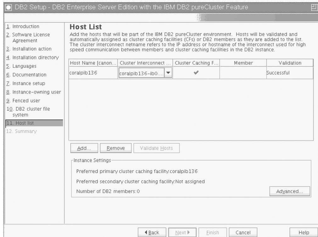
Рисунок 36. Панель Список хостов
