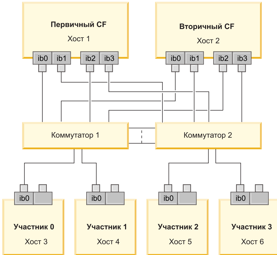
Рисунок 18. 2 CF и четыре участника соединяются с двумя коммутаторами.
