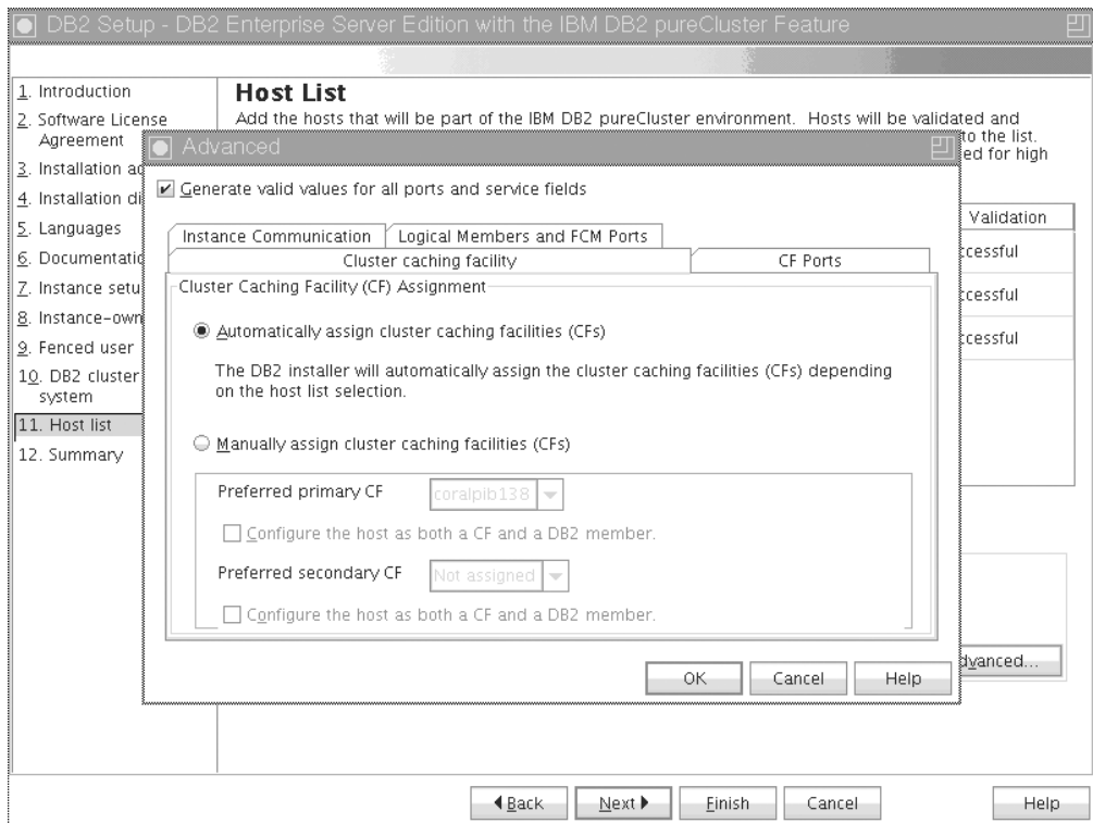
Рисунок 40. Дополнительные параметры экземпляра - вкладка Механизм кэширования кластера
