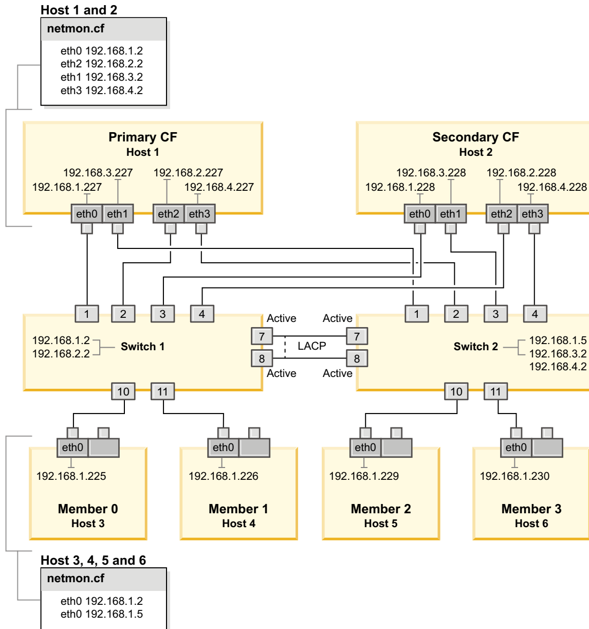
Рисунок 23. Два CF и четыре участника соединяются с двумя коммутаторами.
