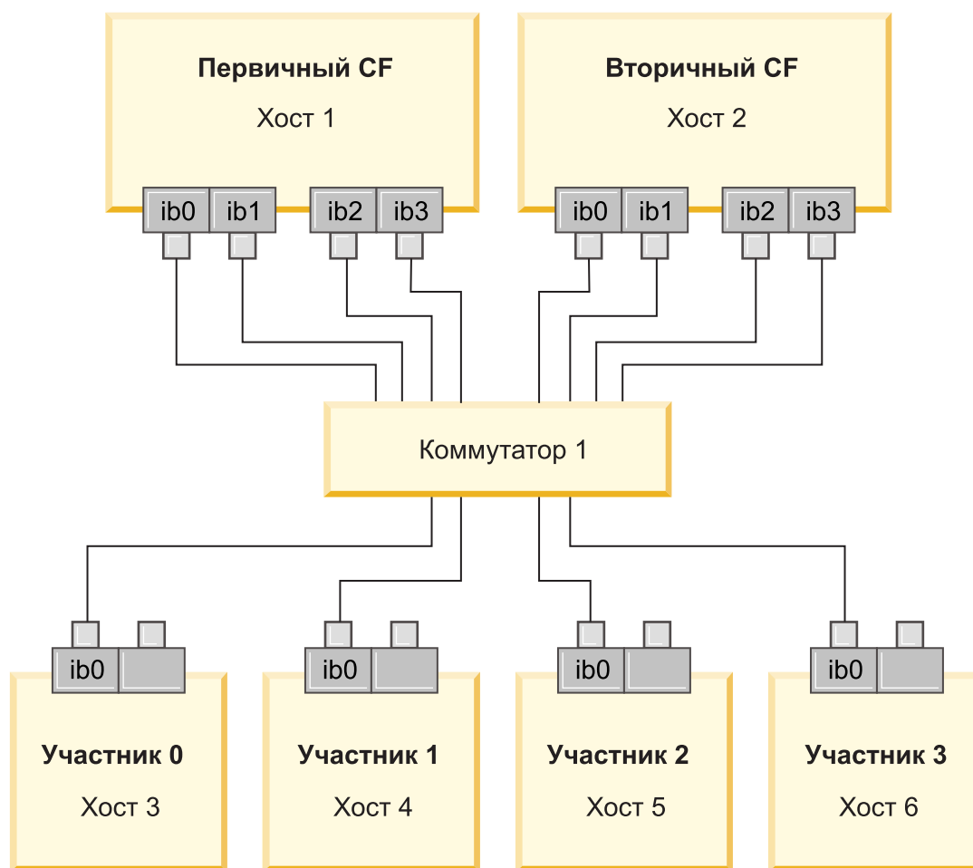
Рисунок 17. 2 CF и четыре участника соединяются с одним коммутатором.
