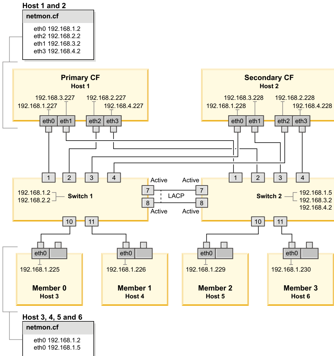
Рисунок 21. Два CF и четыре участника соединяются с двумя коммутаторами.
