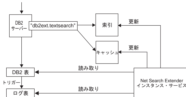
図 5. ストアード・プロシージャ検索の使用
