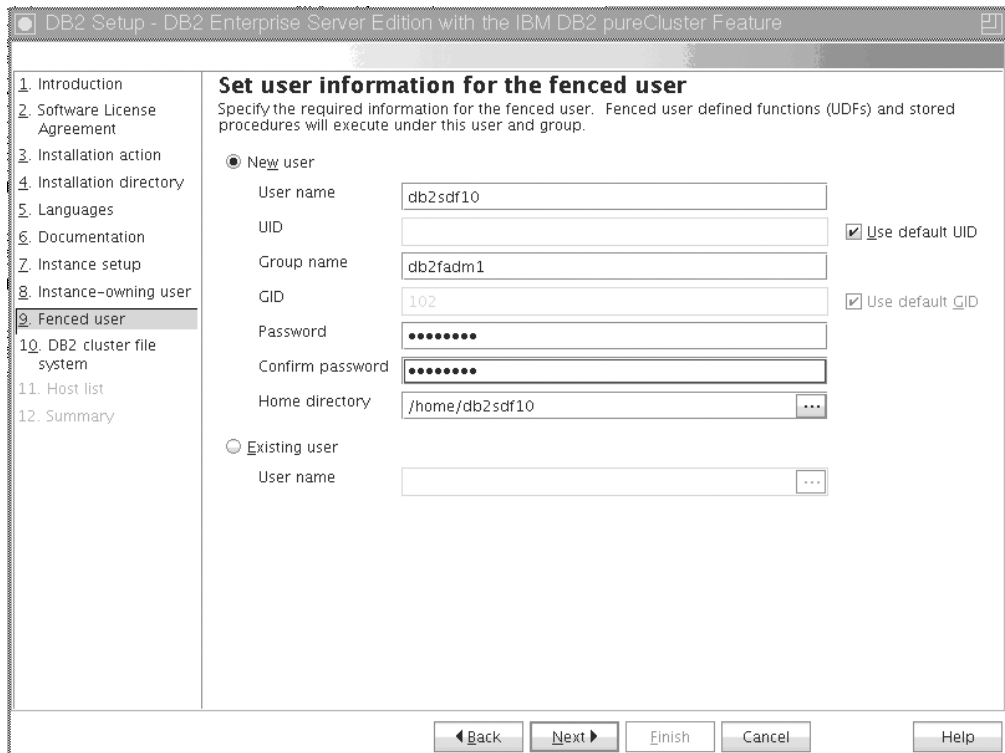
図 34. 「fenced ユーザーのユーザー情報の設定」パネル
