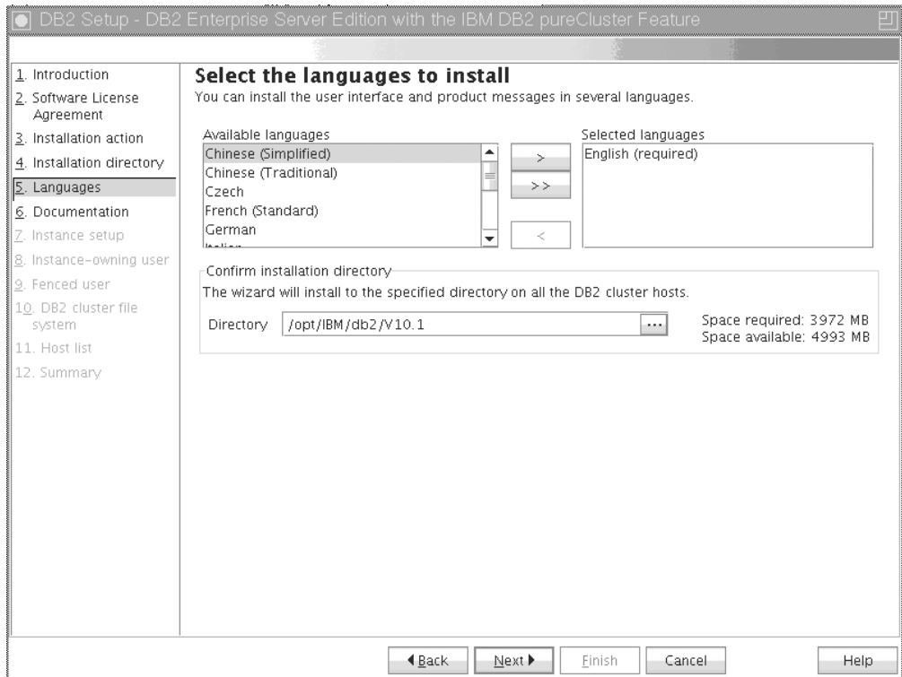
図 30. 「インストールする言語の選択」パネル
