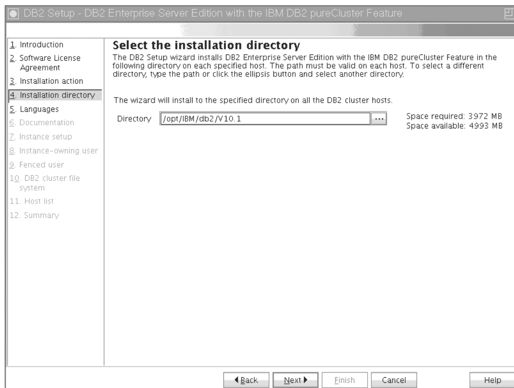
図 29. 「インストール・ディレクトリーの選択」パネル
