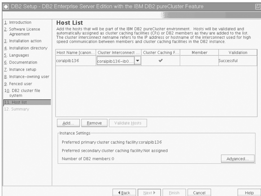
図 36. 「ホスト・リスト」パネル
