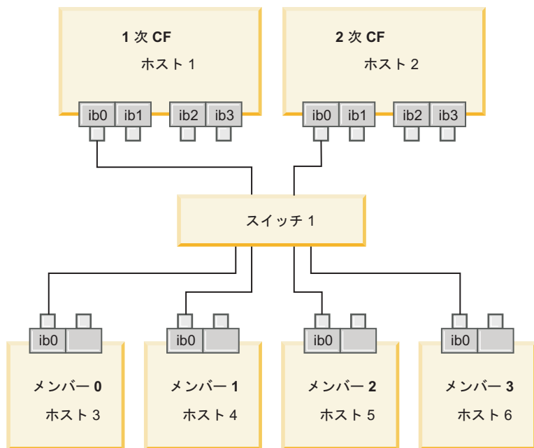
図 19. 2 つの CF と 4 つのメンバーが 1 つのスイッチに接続しています。
