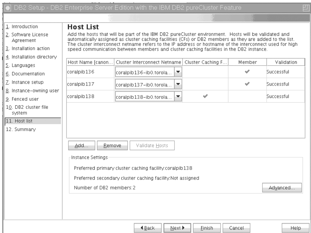
図 39. ホストが 3 つ (1 つはプリロードされた IIIH 、2 つは追加されたホスト) の「ホスト・リスト」パネル
