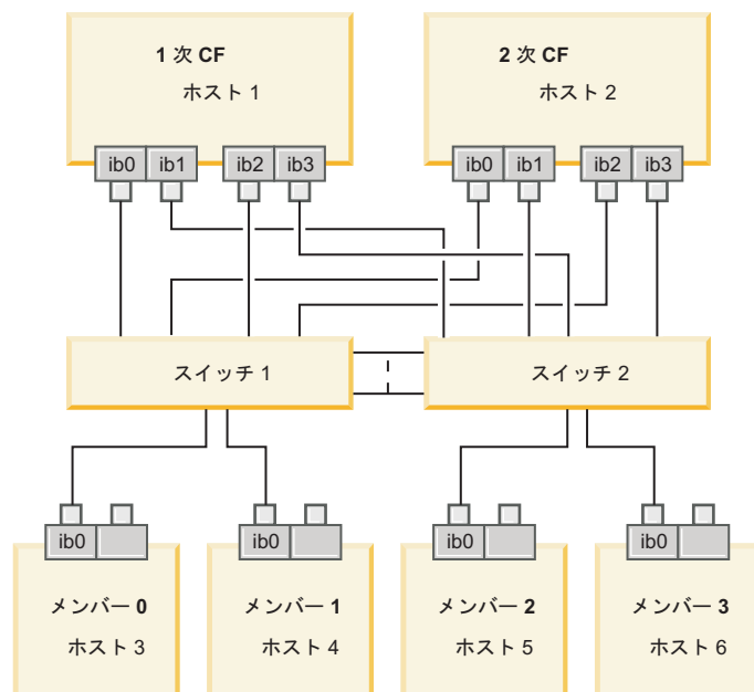
図 18. 2 つの CF と 4 つのメンバーが 2 つのスイッチに接続しています。
