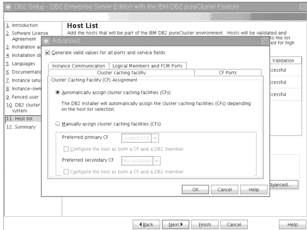
図 40. 「拡張インスタンス設定 (Advanced Instance Settings)」 - 「クラスター・キャッシング・ファシリティ」タブ
