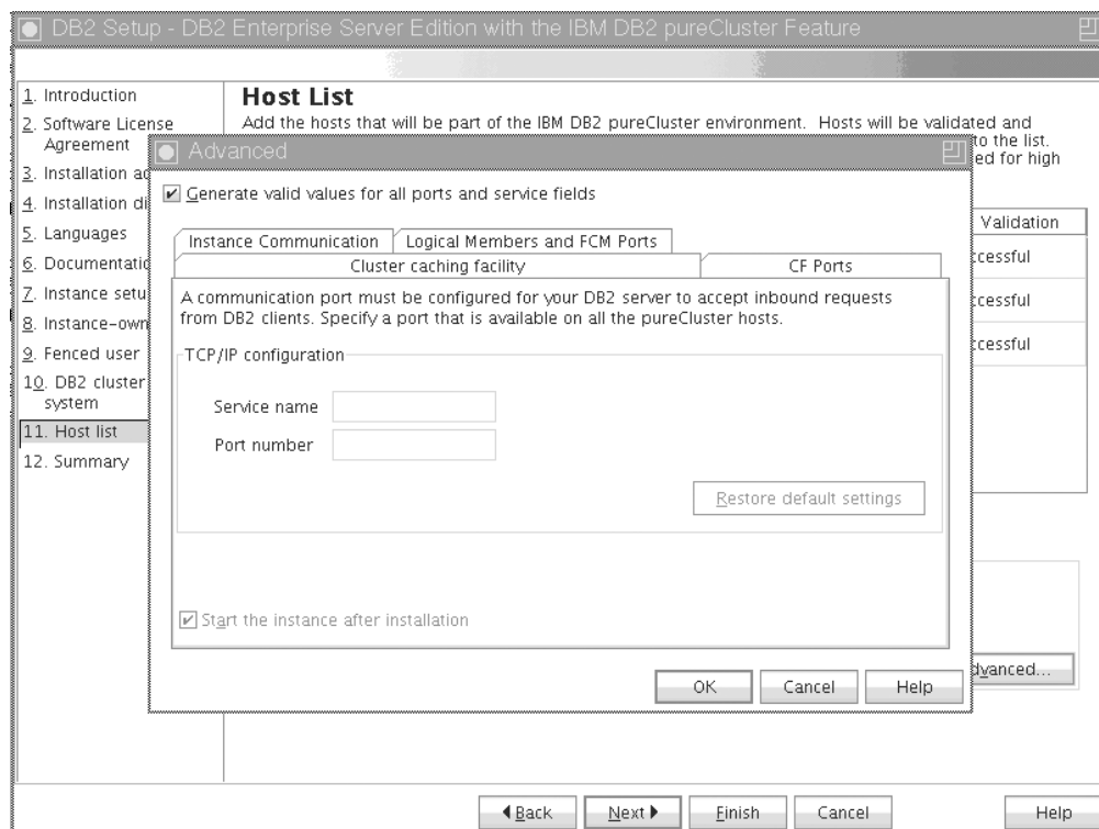
図 42. 「拡張インスタンス設定 (Advanced Instance Settings)」 - 「インスタンス通信」タブ
