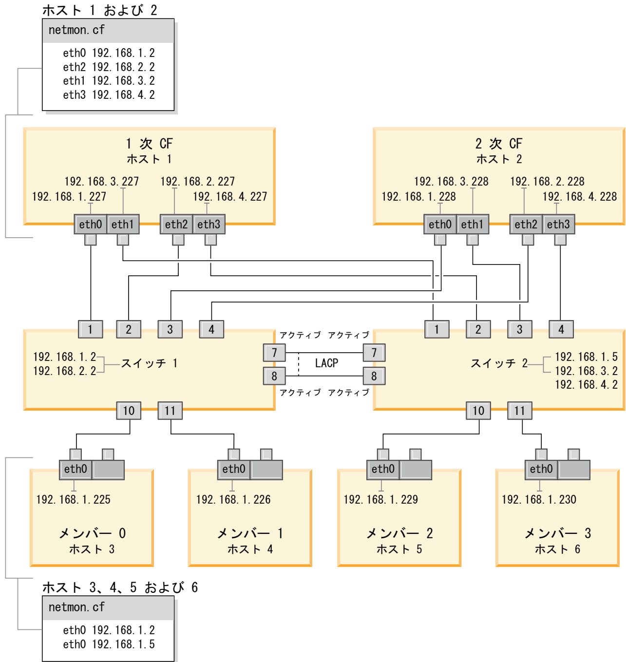
図 21. 2 つの CF と 4 つのメンバーが 2 つのスイッチに接続しています。
