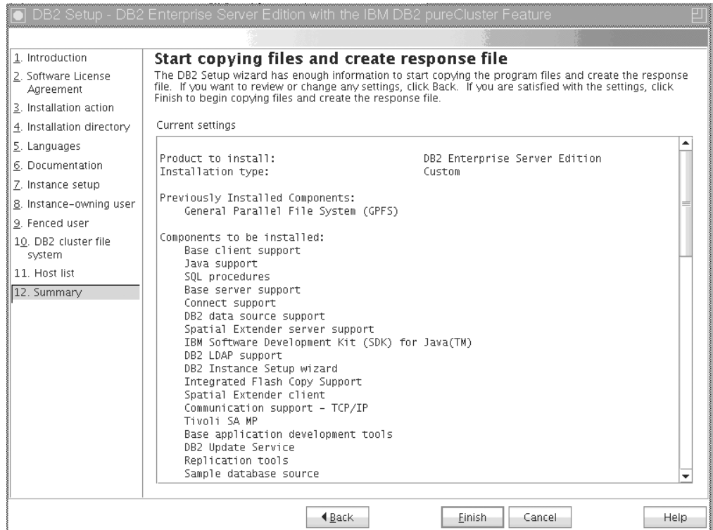
図 44. 「サマリー」 パネル
