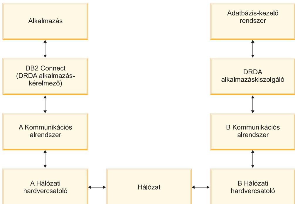
10. ábra: Adatfolyamok DB2 Connect alkalmazása során
