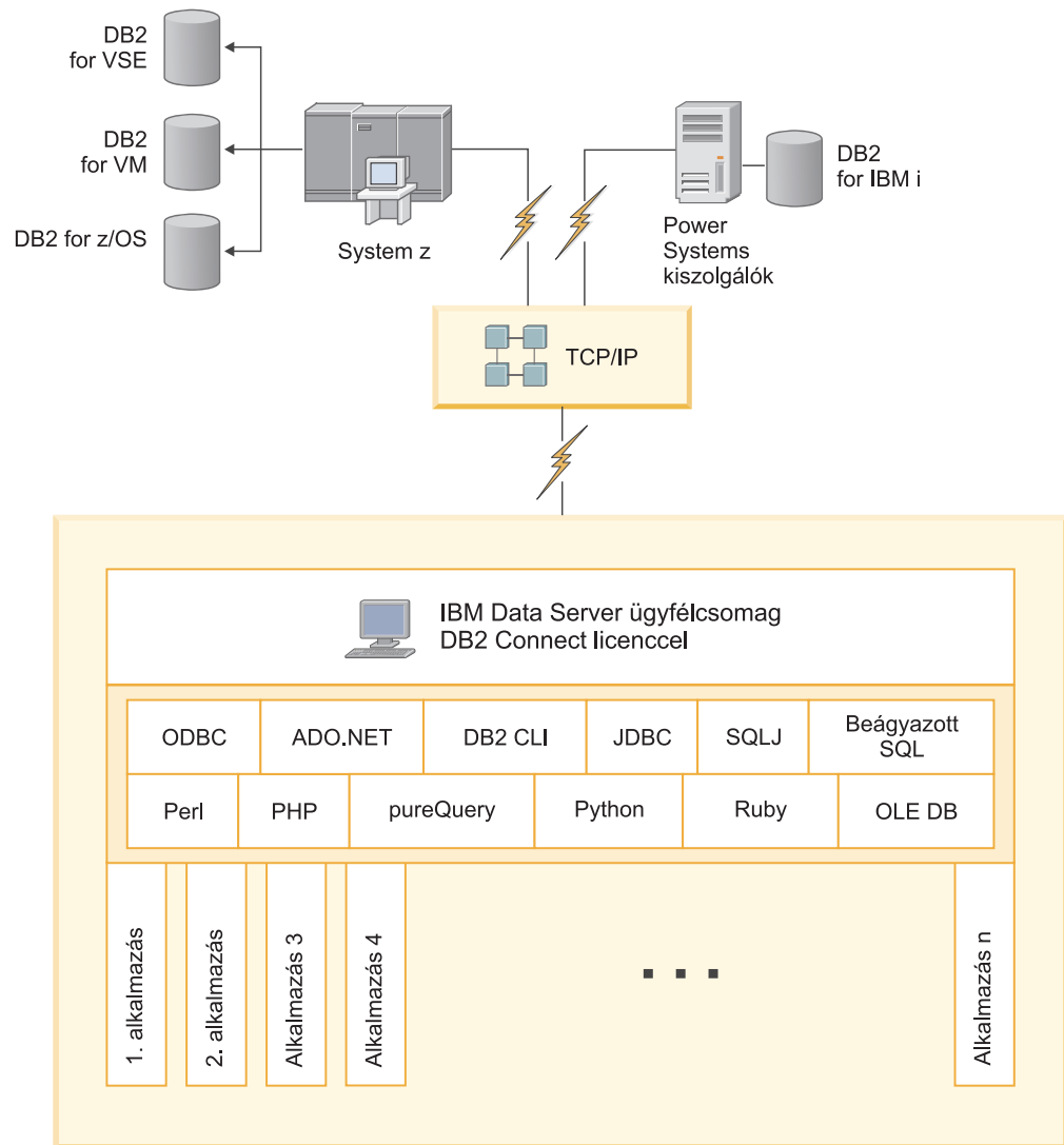
1. ábra: Közvetlen kapcsolat a DB2 Connect és az IBM nagyszámítógépes adatbázis-kiszolgáló között
