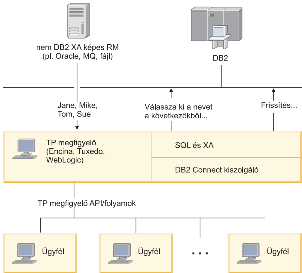
3. ábra: DB2 Connect támogatás TP figyelőkhöz
