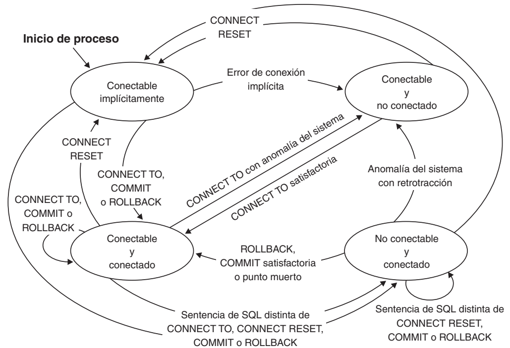
Figura 9. Transiciones del estado de conexión si la conexión implícita está disponible
