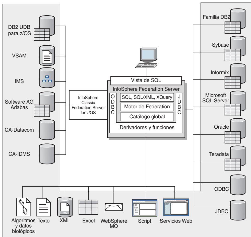
Figura 12. Componentes de un sistema federado
