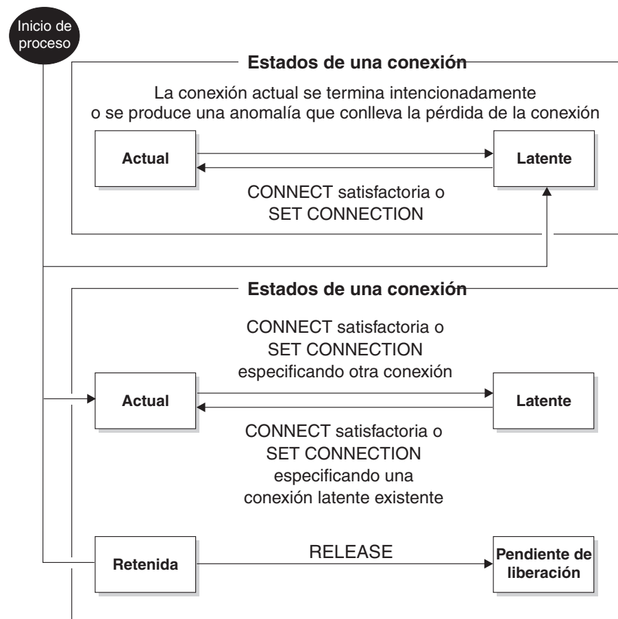
Figura 11. Transiciones del estado de las conexiones de las unidades de trabajo distribuidas dirigidas por aplicación
