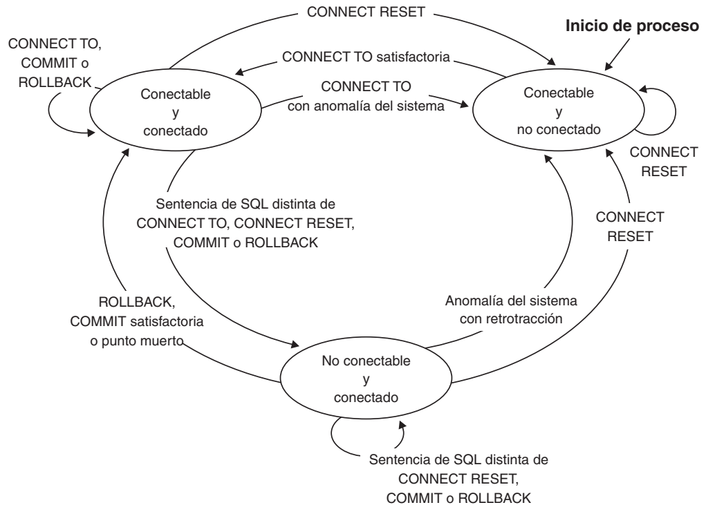
Figura 10. Transiciones del estado de conexión si la conexión implícita no está disponible
