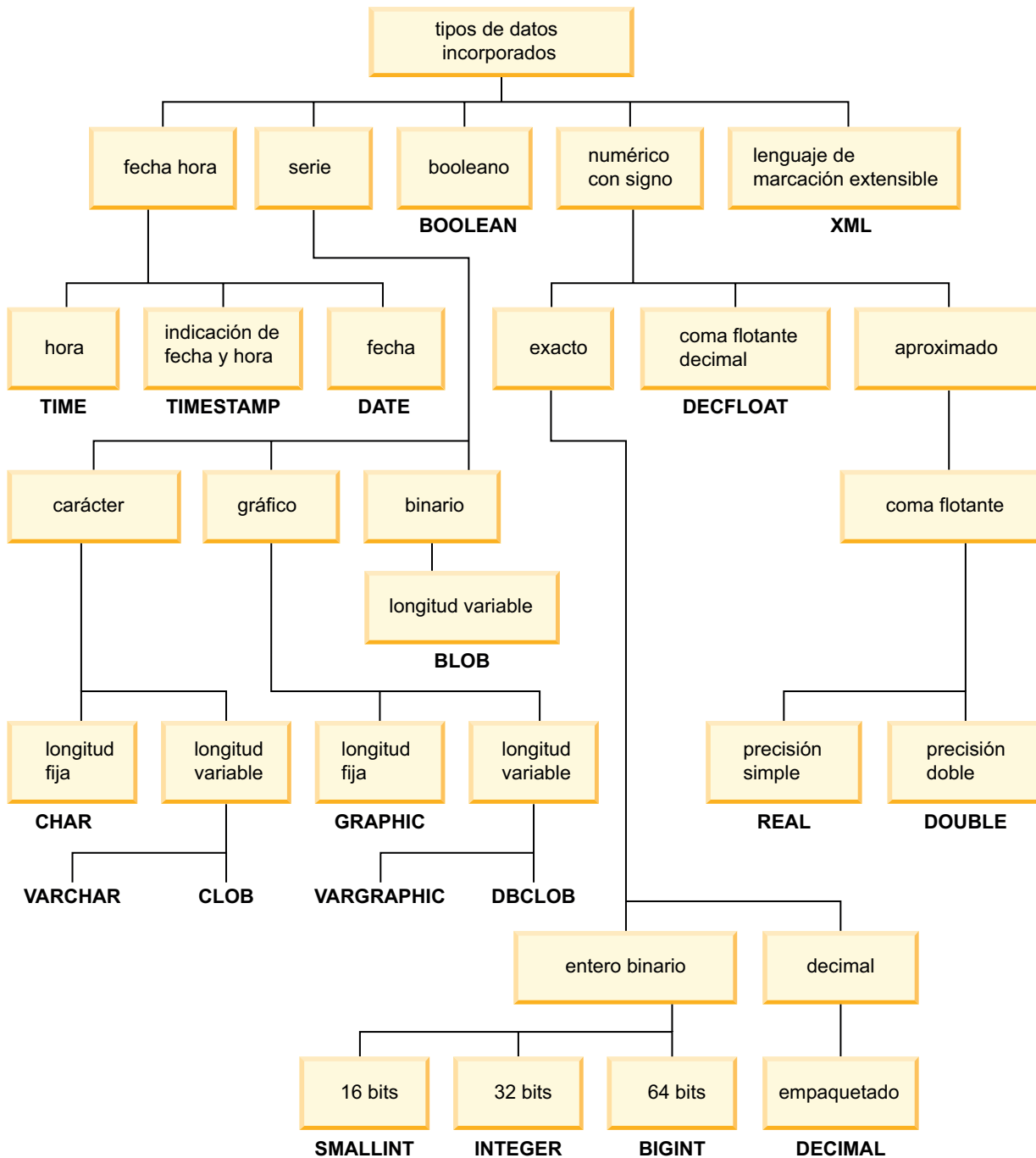
Figura 13. Tipos de datos internos de DB2 soportados
