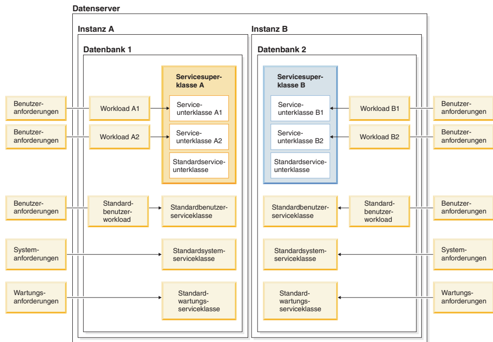
Abbildung 41. Datenserverkonfiguration: Mehrere DB2-Instanzen
