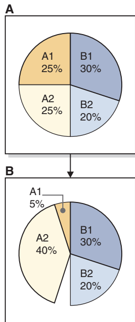
Abbildung 44. CPU-Grenzwert und mehrere DB2-Instanzen: Szenario 3
