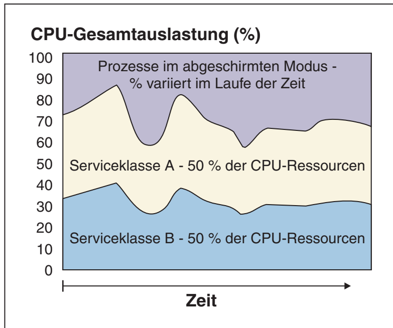
Abbildung 23. Prozentsatz der CPU-Gesamtauslastung
