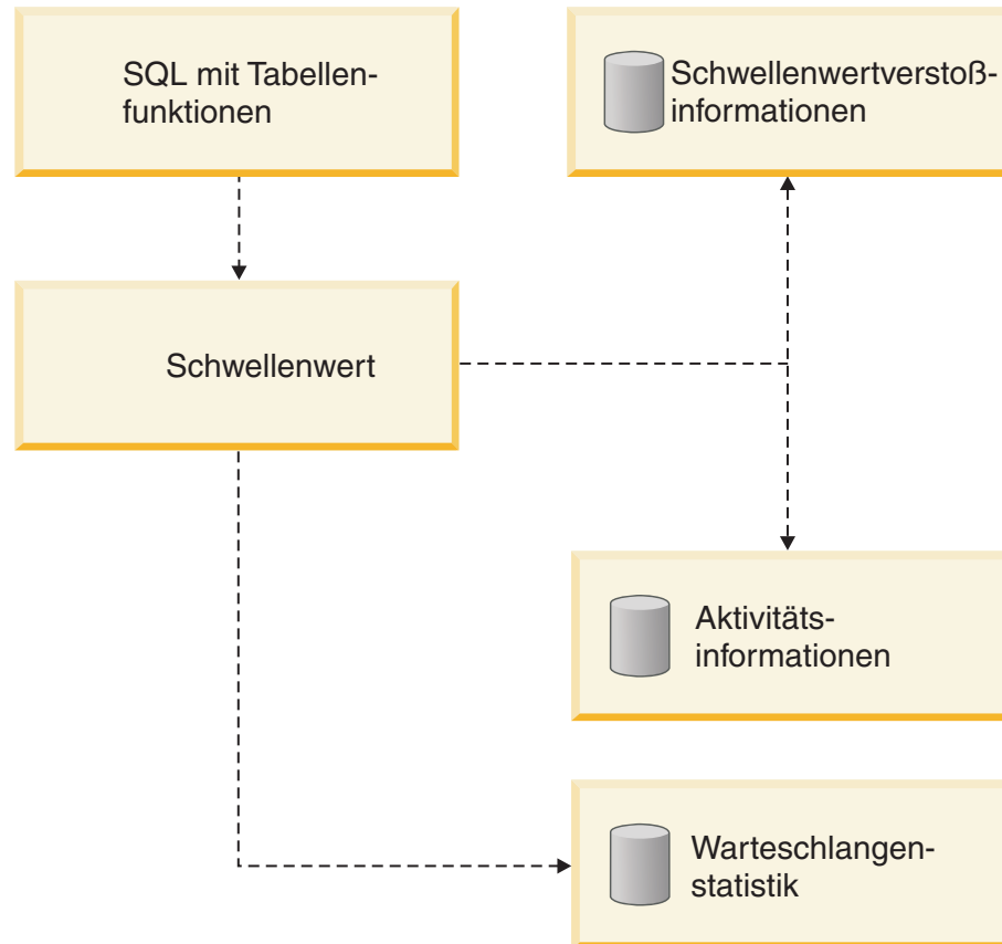
Abbildung 50. Für Schwellenwerte verfügbare Überwachungsdaten
