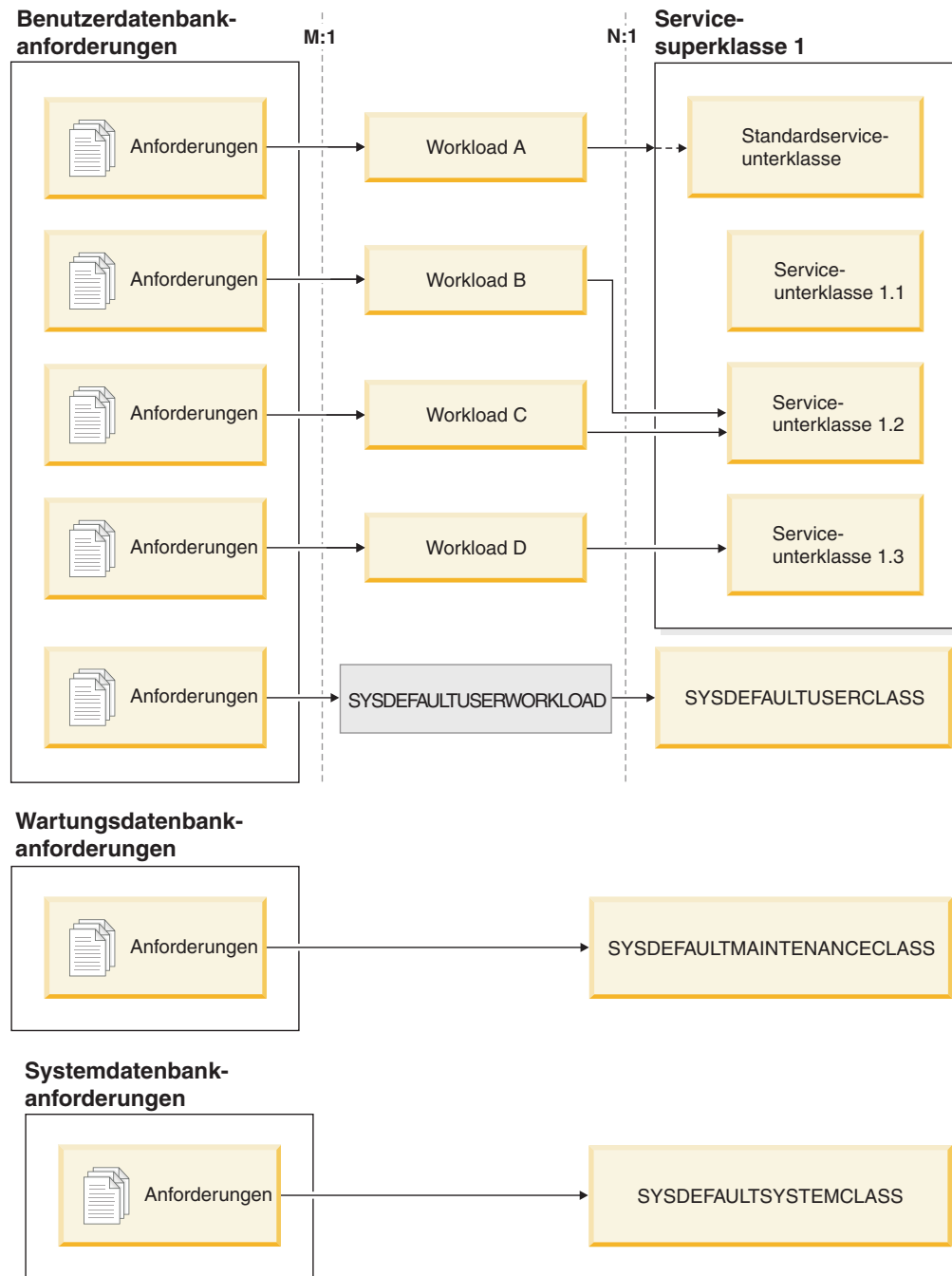
Abbildung 14. Datenbankverbindungen, die einer Servicesuperklasse zugeordnet sind
