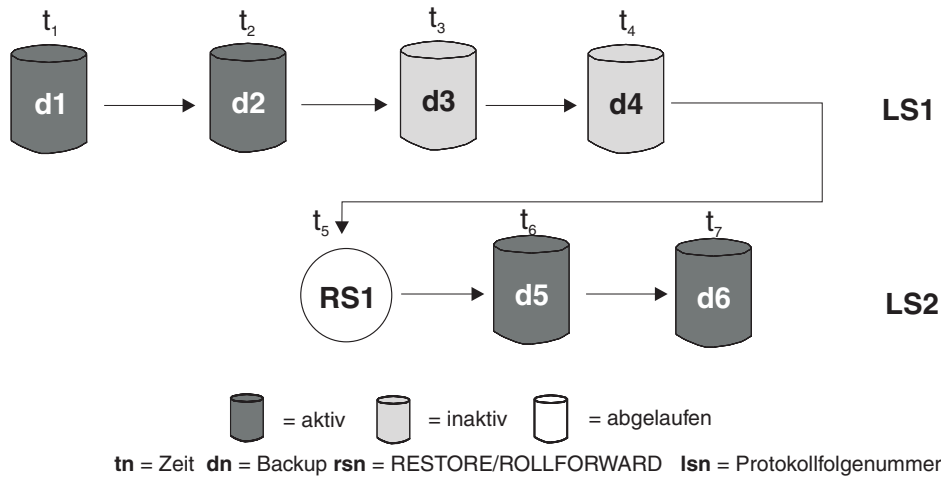
Abbildung 14. Inaktive Datenbankbackups
