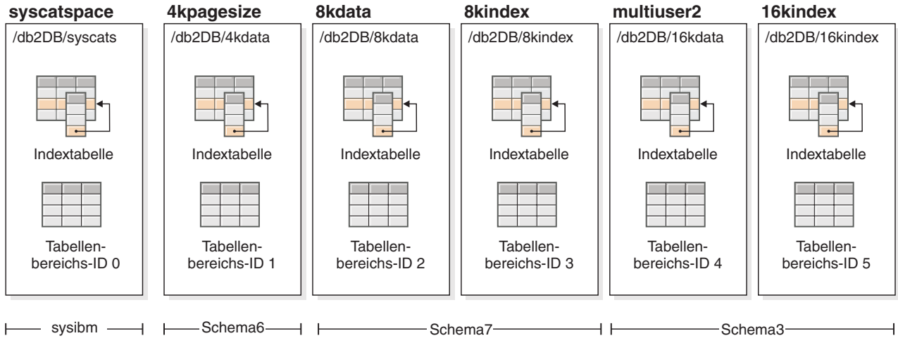
Abbildung 27. Datenbank TARGETDB
