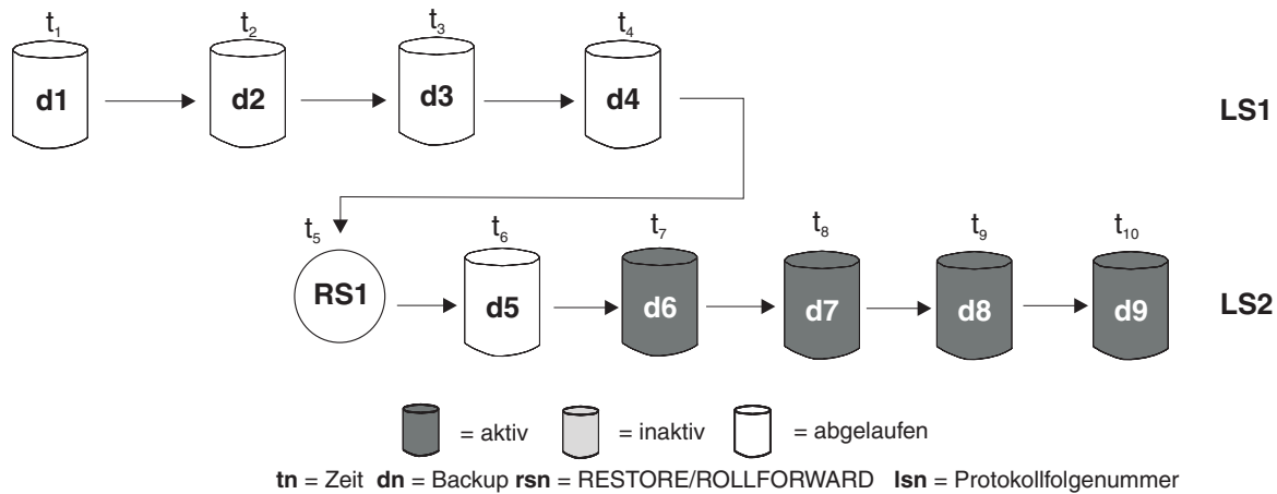
Abbildung 17. Abgelaufene Protokollfolge
