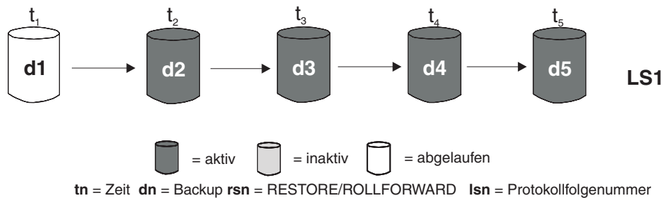
Abbildung 15. Abgelaufene Datenbankbackups
