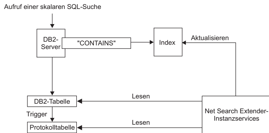
Abbildung 4. Ausführung von Suchoperationen mit einer skalaren SQL-Suchfunktion
