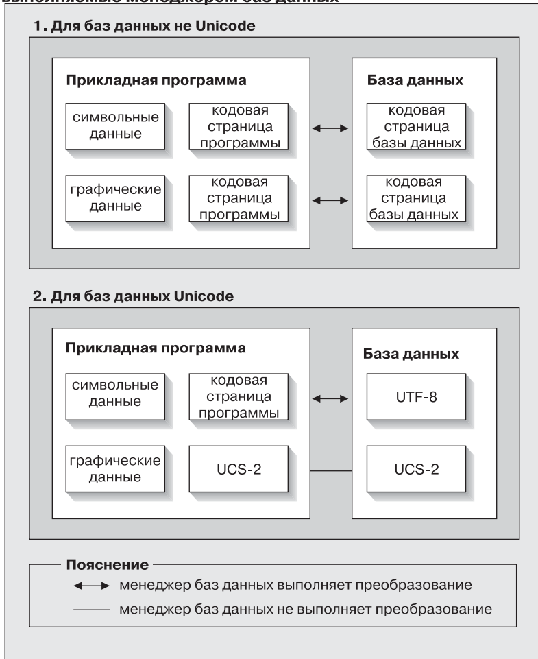
Рисунок 1. Преобразования кодовых страниц, выполняемые менеджером баз данных
