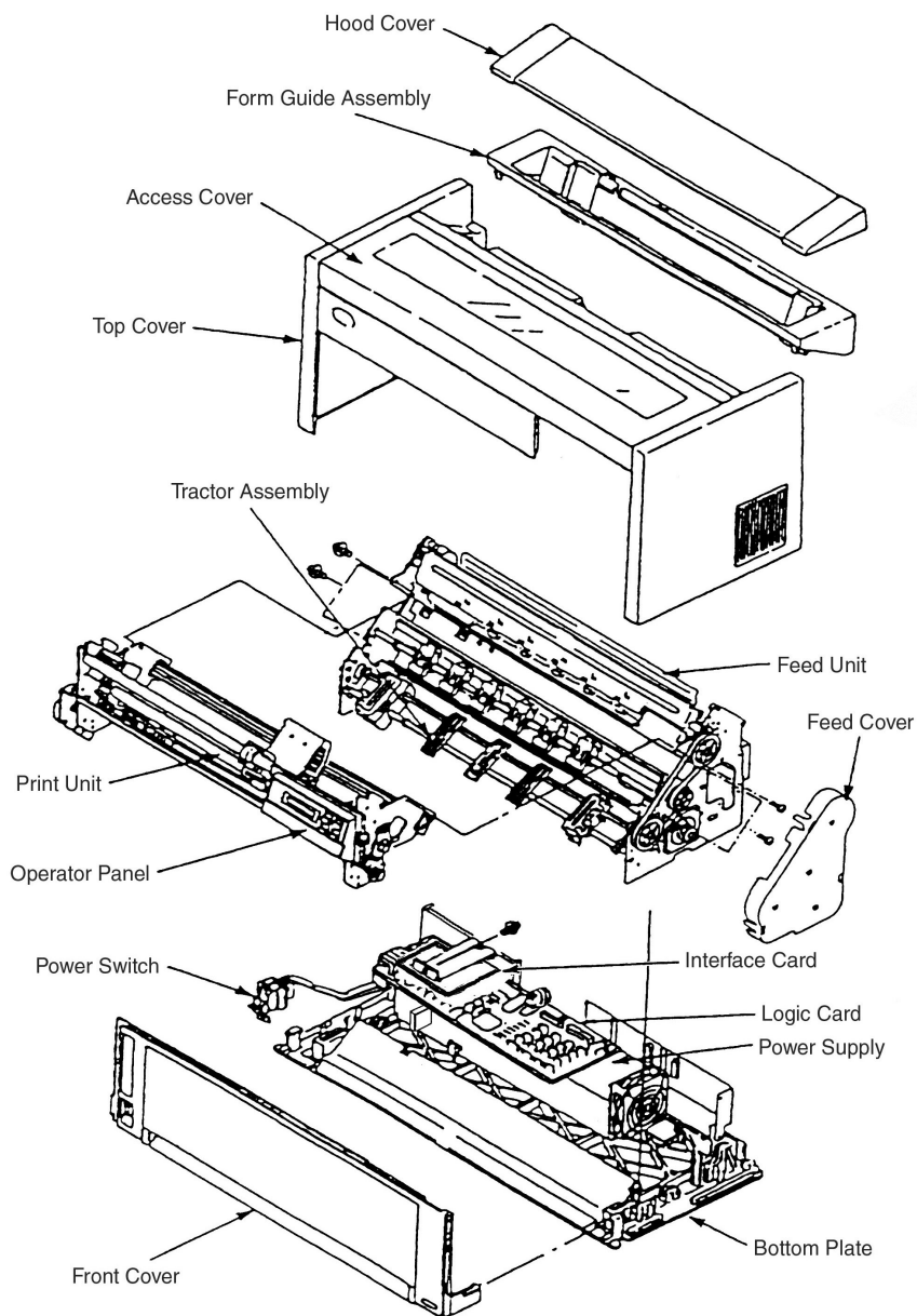
図4-1 InfoPrint 5579シリアル・プリンターの主要部品配置図
