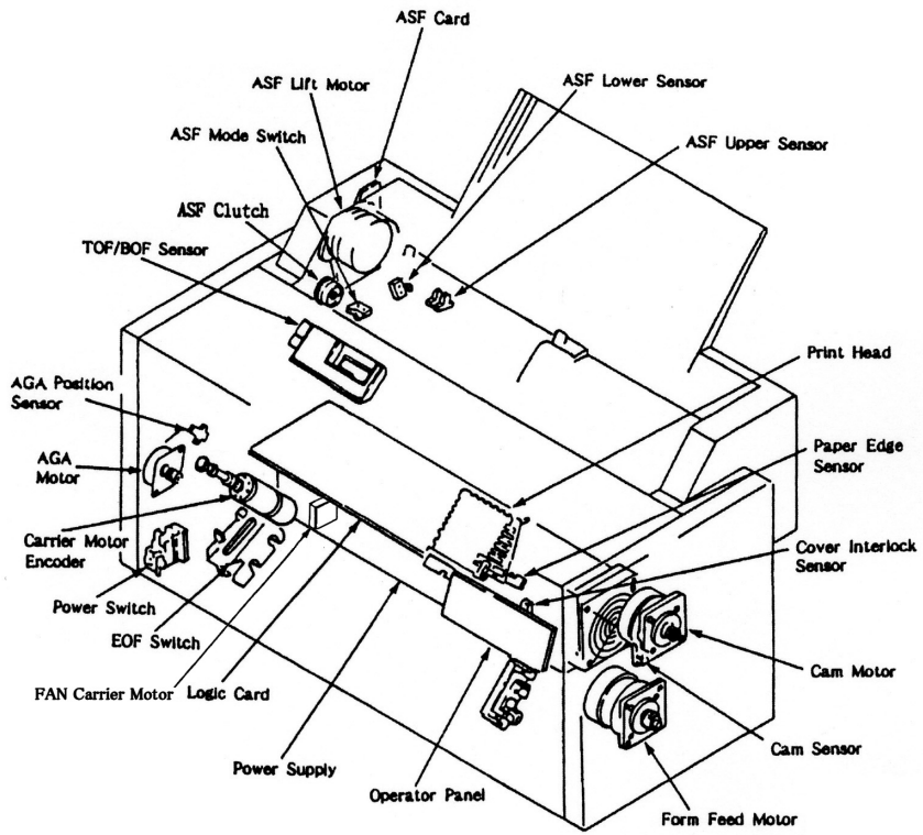
図4-2 電気部品配置図
