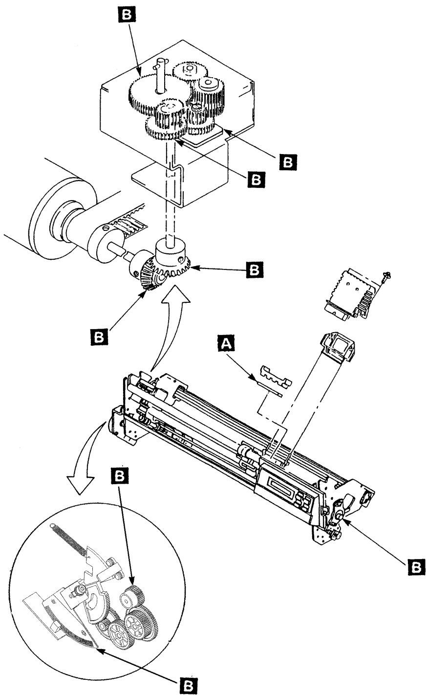
図 8-2 (2/2). IBM 5577-W02 の注油個所と油の種類
