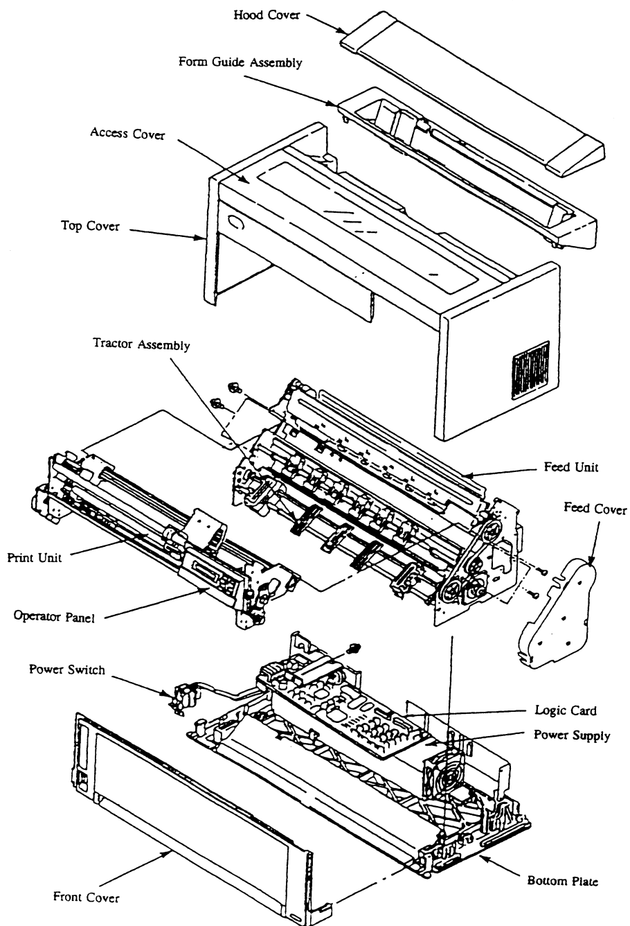
図 5-1. IBM 5577-V02 シリアル・プリンターの主要部品配置図
