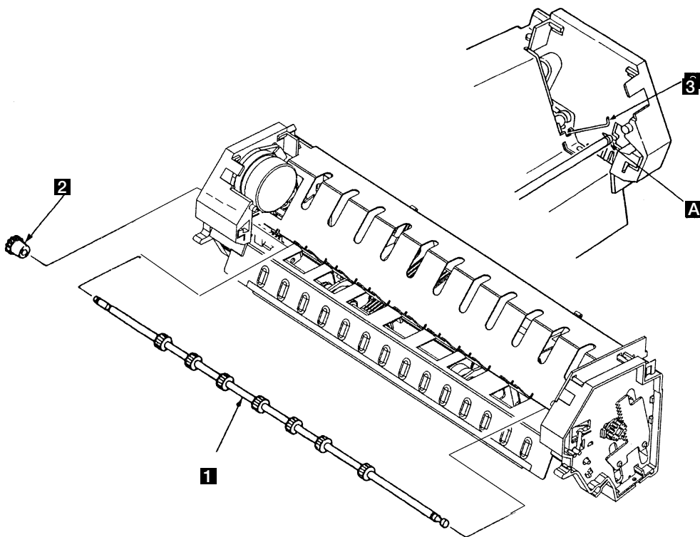
図 6-36. ASF Stacker Roll
