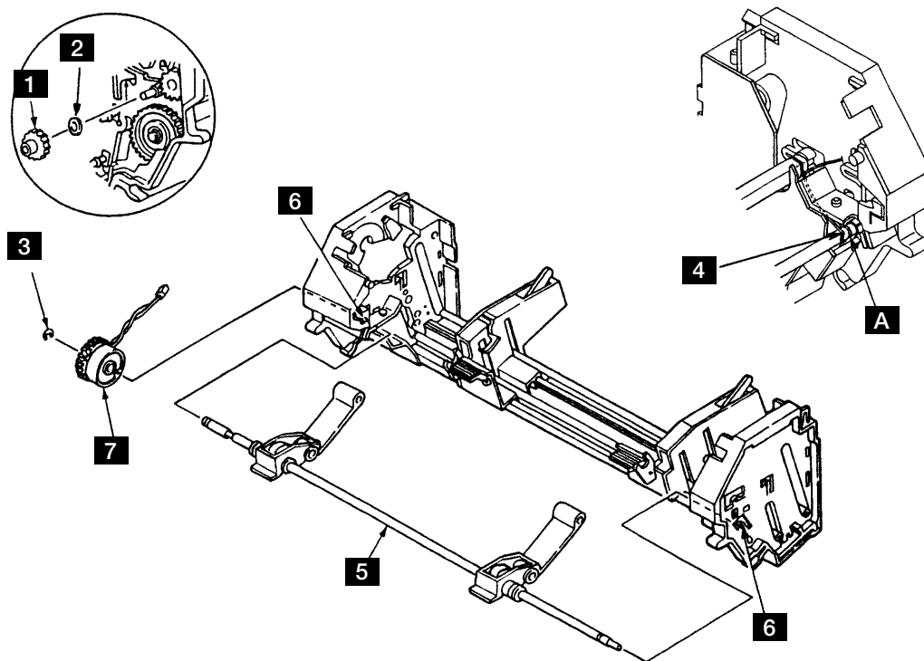
図 6-40. ASF Feed Roll Assembly と Clutch Assembly
