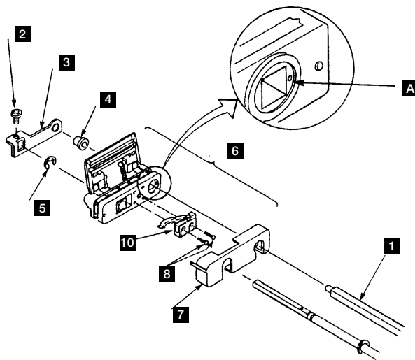
図 6-27. EOF Switch
