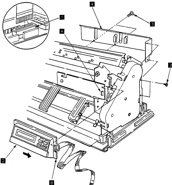
図 6-4. Operator Panel
