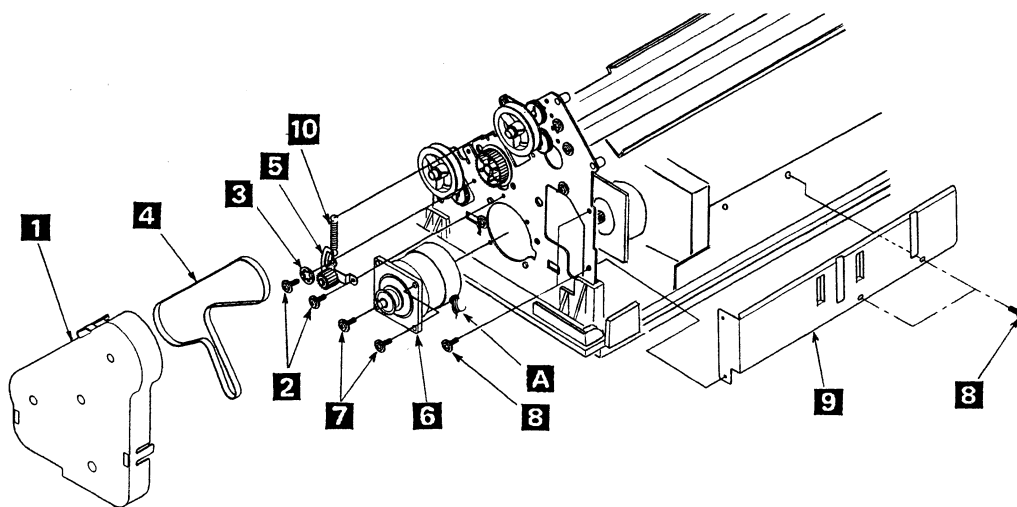
図 6-18. Feed Motor
