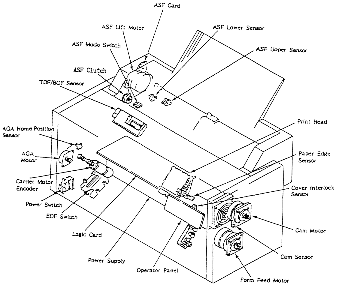
图 5-2. 电气部品配置图
