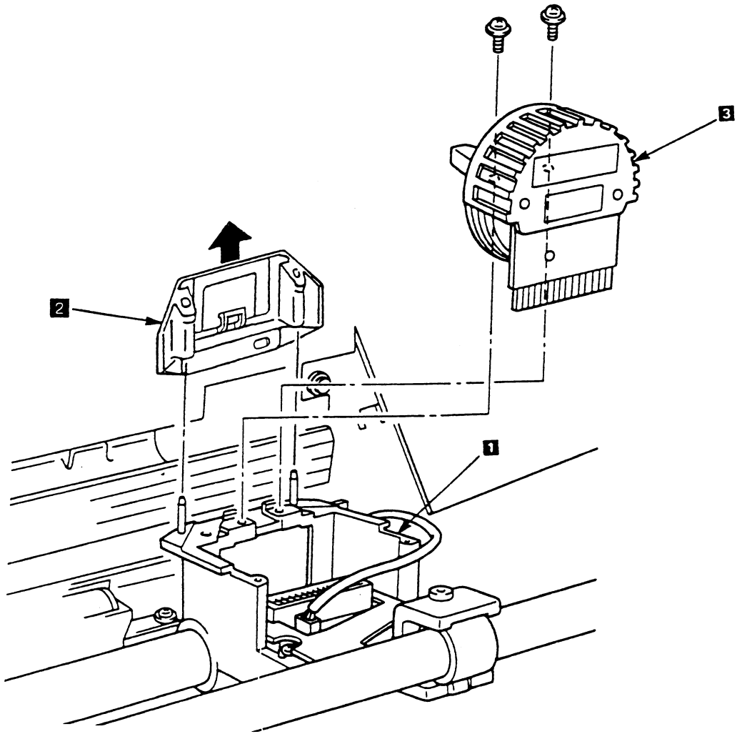
図 6-8. Ribbon Shield
