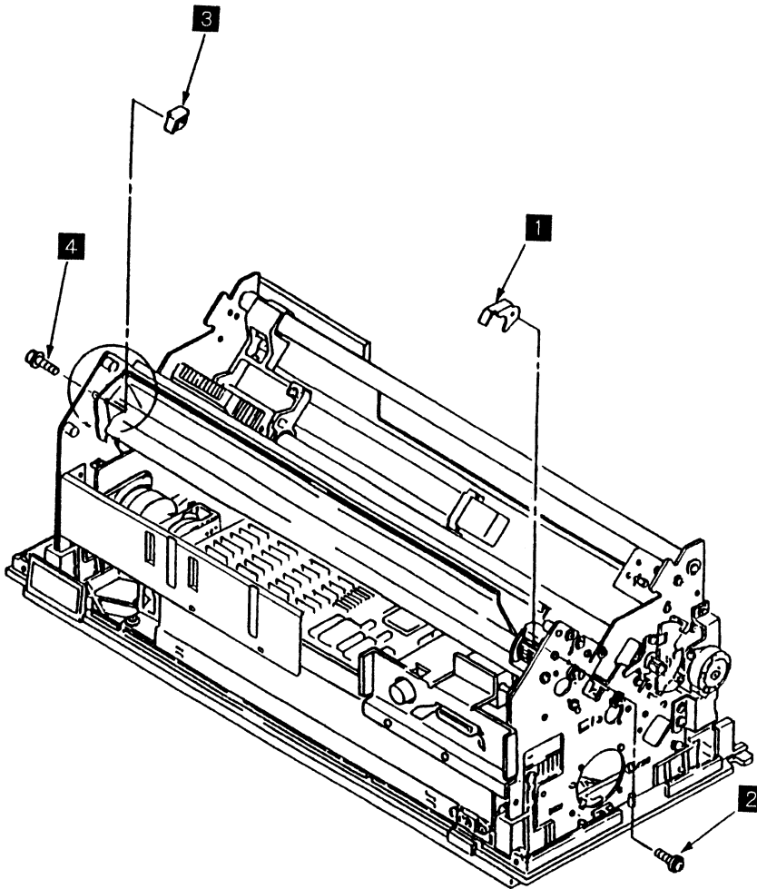
図 6-12. ASF Guide Bracket
