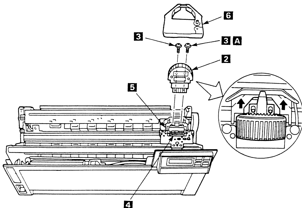
図 6-7. Print Head
