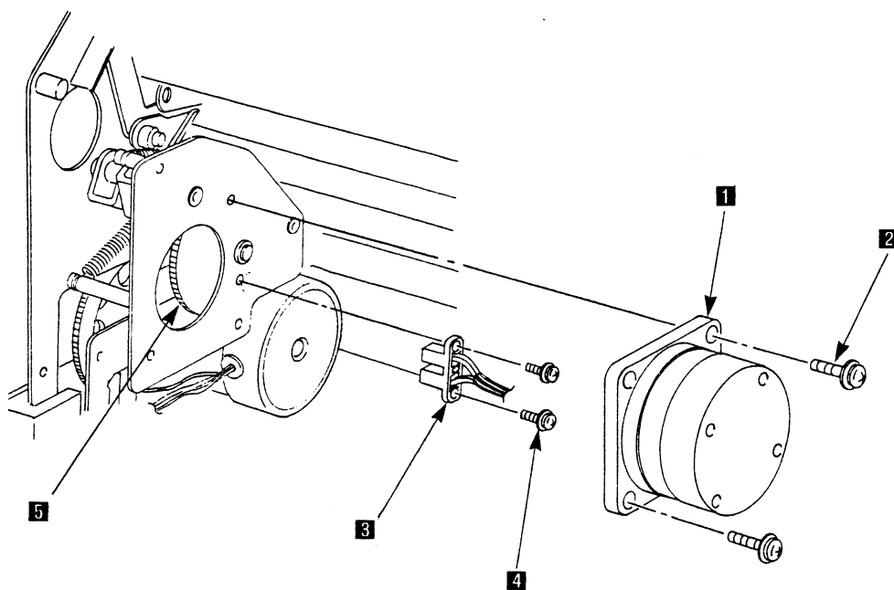
図 6-28. Cam Motor と Cam Sensor
