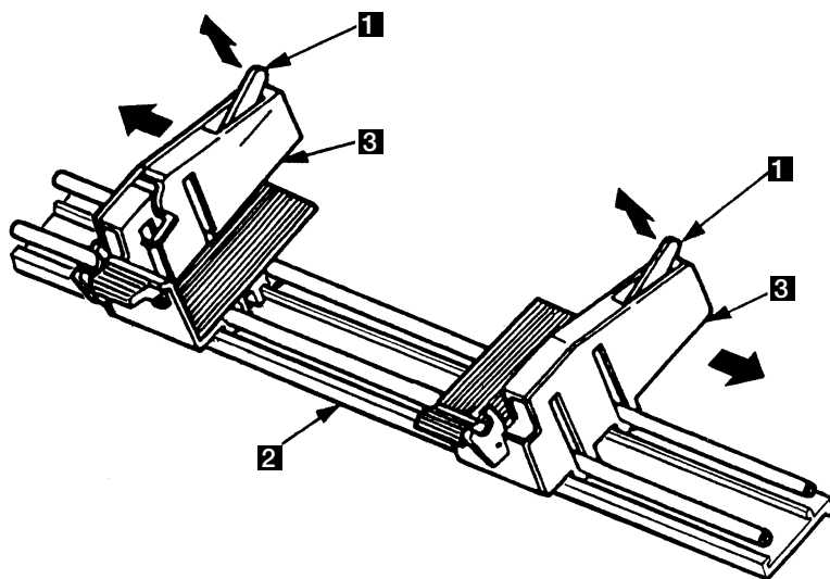
図 6-43. ASF Hopper Guide Assembly
