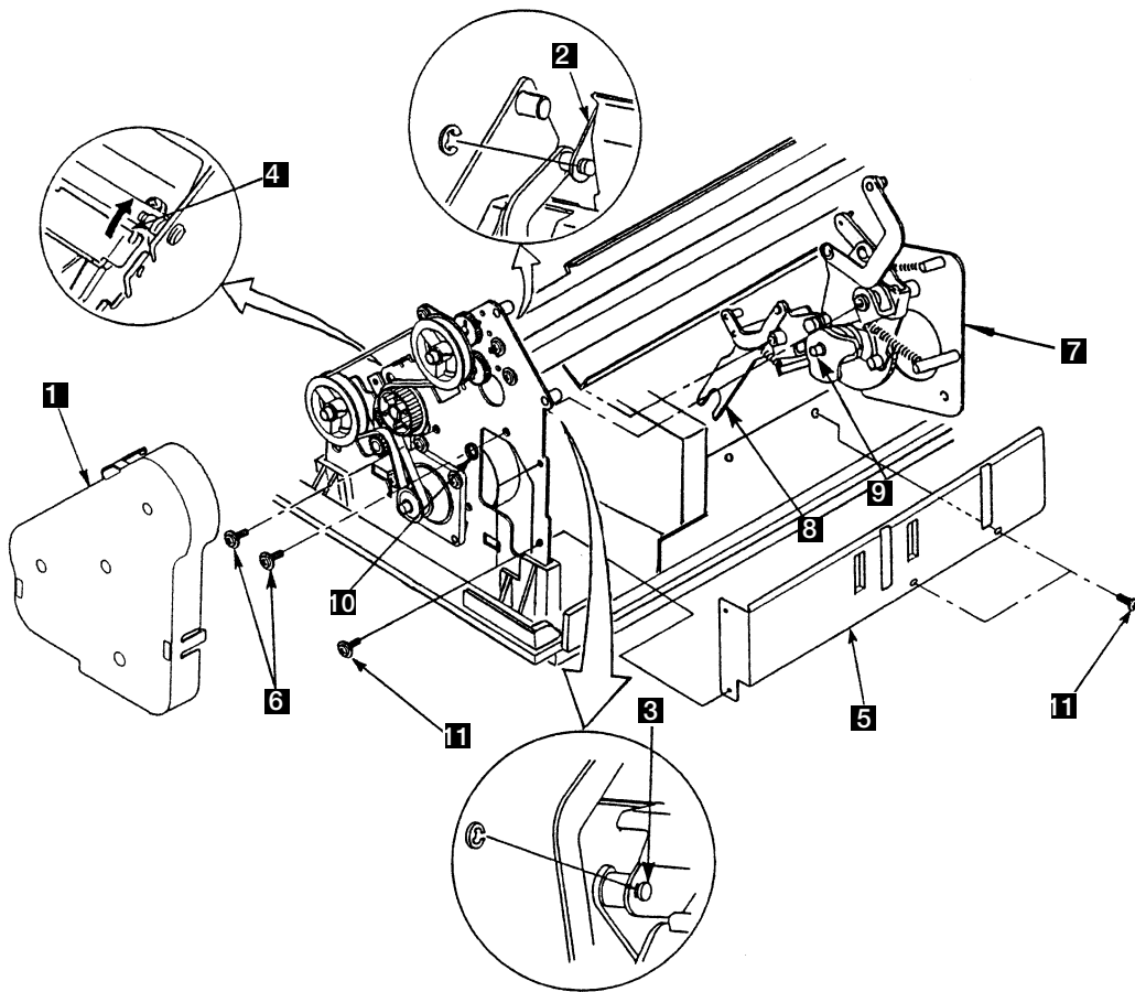
図 6-29. Cam Assembly
