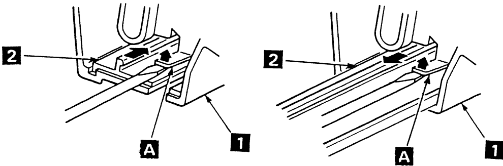
図 6-42. ASF Left/Right Side Frame
