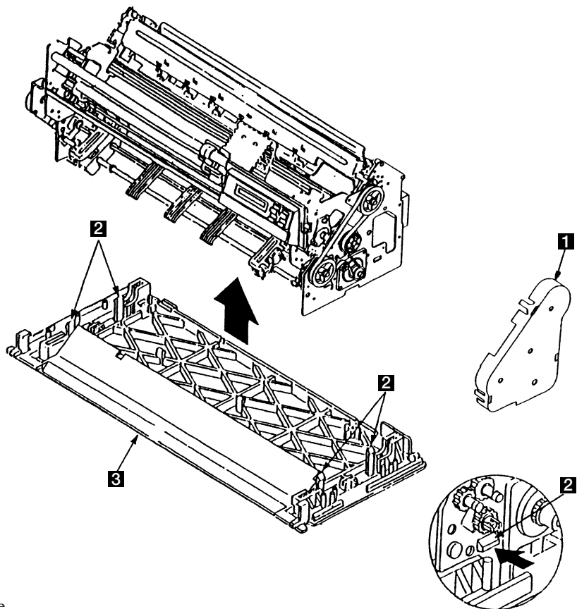
図 6-30. Bottom Plate
