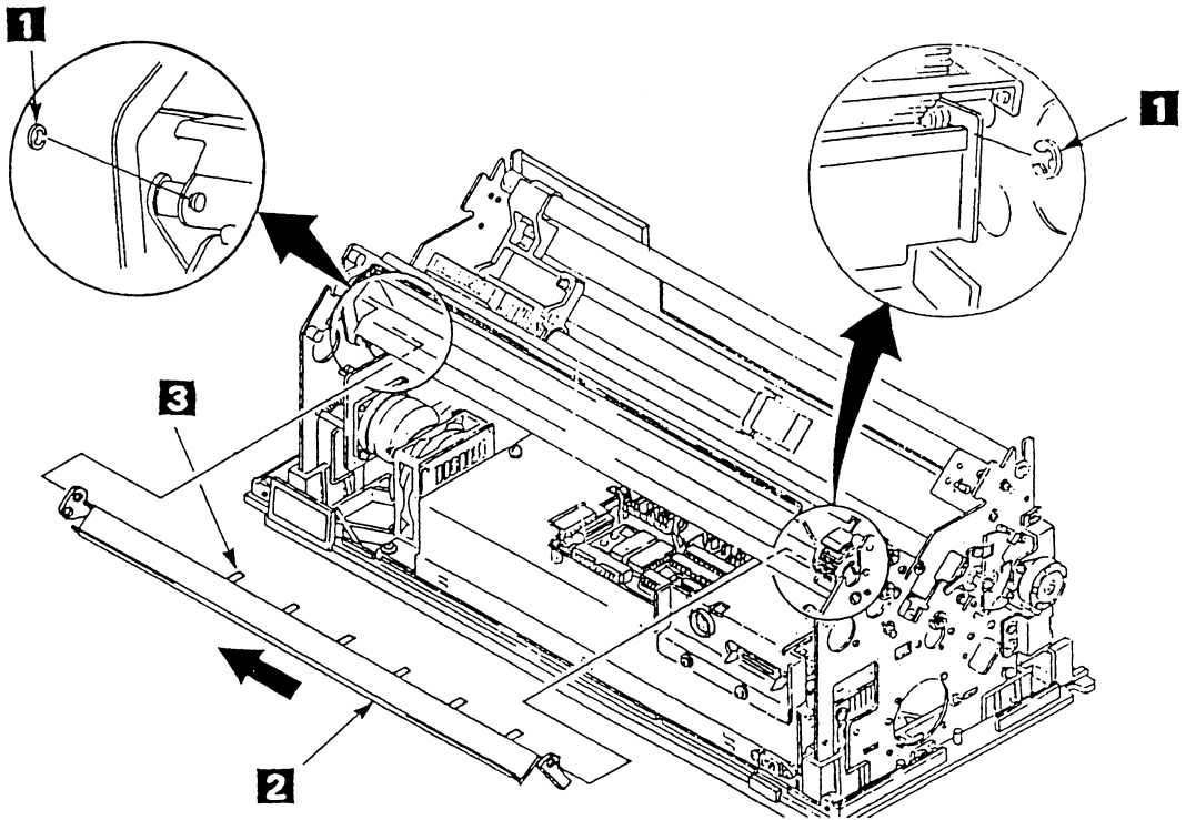
図 6-21. Stopper Plate
