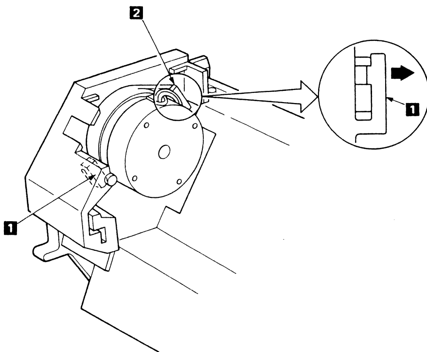
図 6-37. ASF Lift Motor
