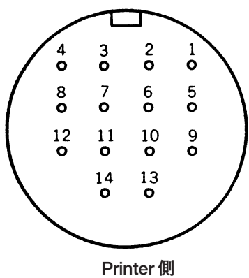
図 5-6. ASF コネクター J14(ASF)
