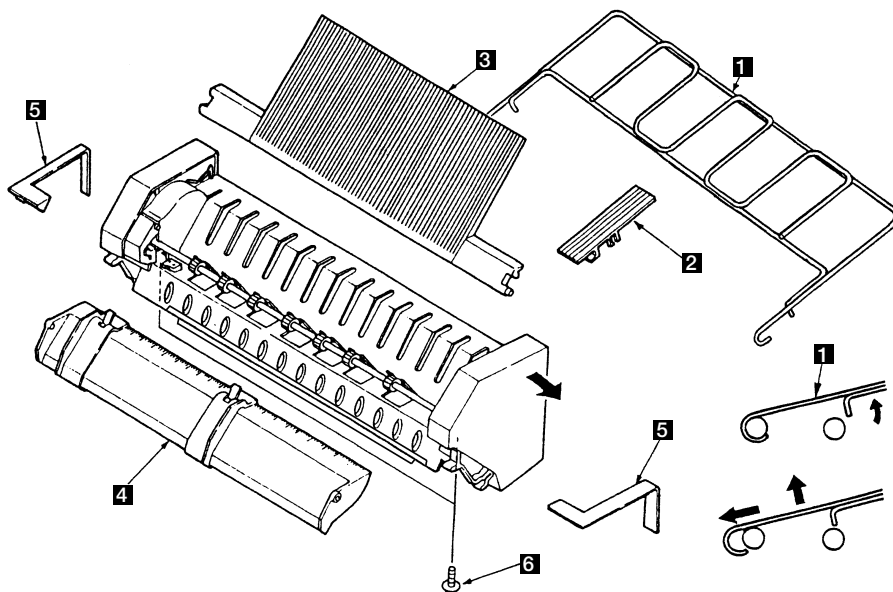
図 6-32. ASF Guide Plate
