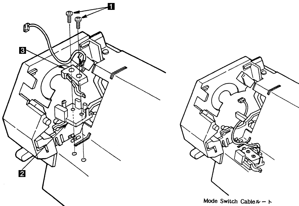
図 6-38. ASF Mode Switch と Stacker Spacer
