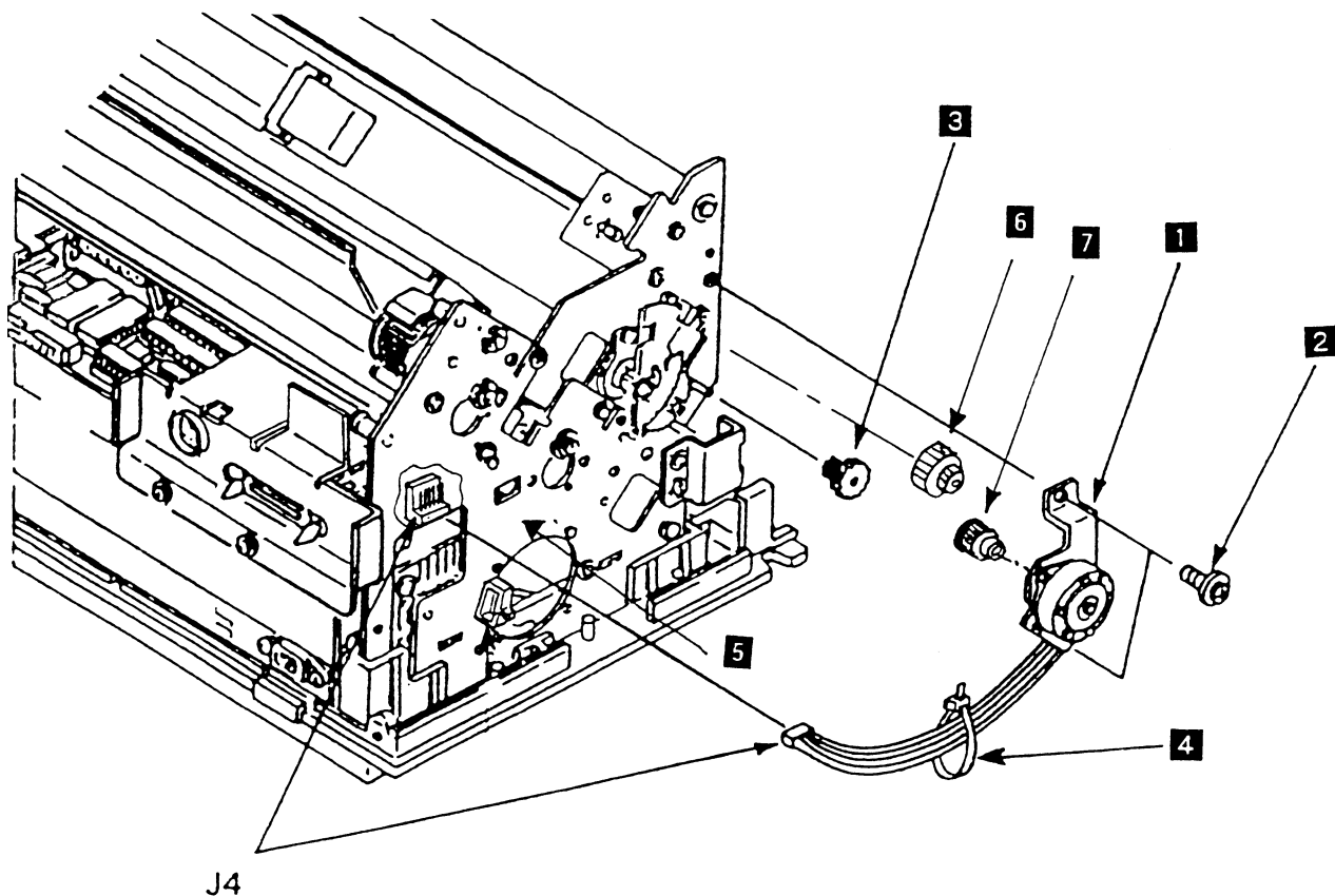
図 6-11. AGA Motor Assembly と Idler Gear
