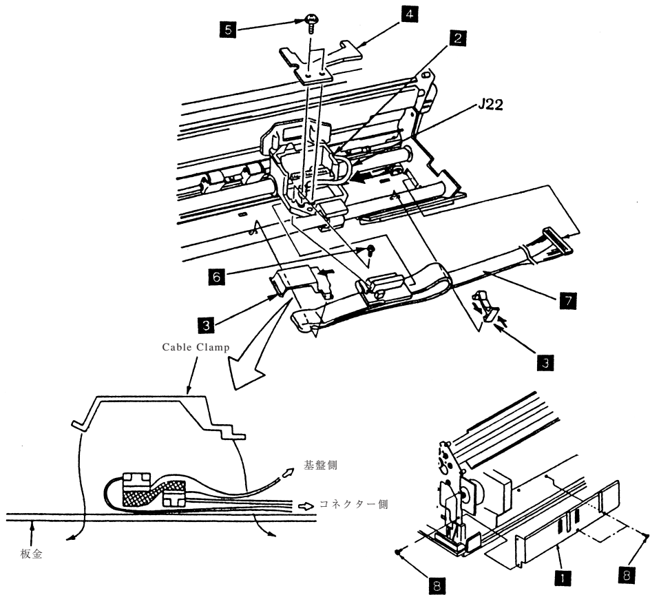
図 6-9. Print Head Cable
