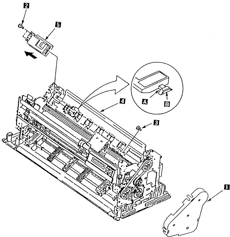
図 6-25. TOF/BOF Sensor
