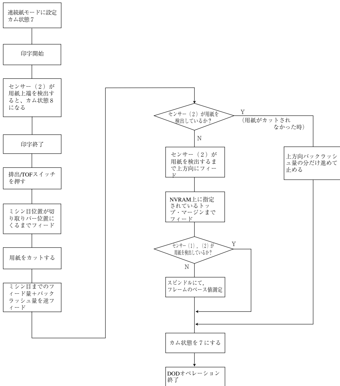
図 2-14. DODハンドリング・フローチャート
