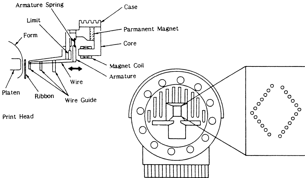
図 2-2. プリント・ヘッド
