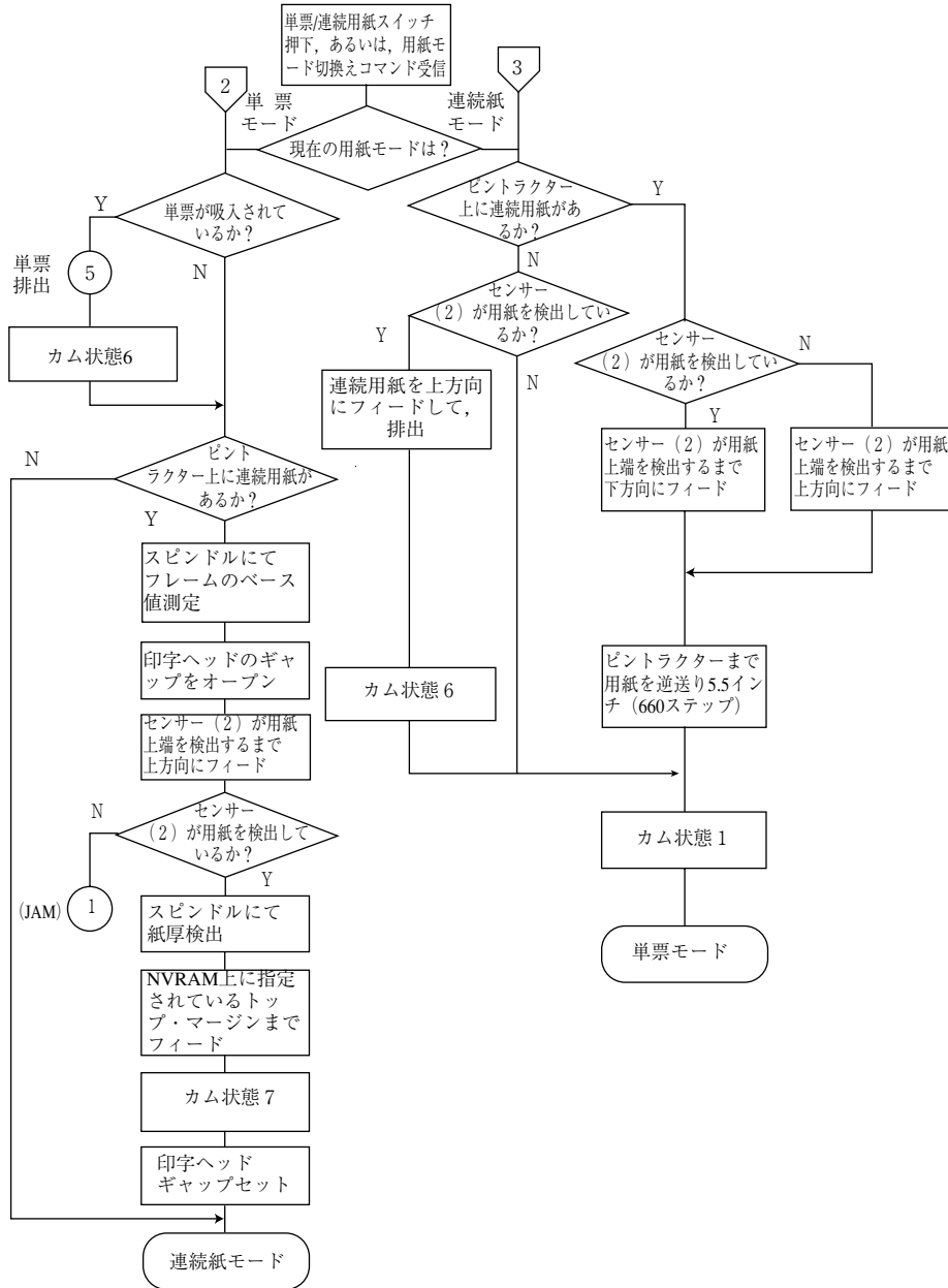
図 2-11. 用紙モード切り換えフローチャート
