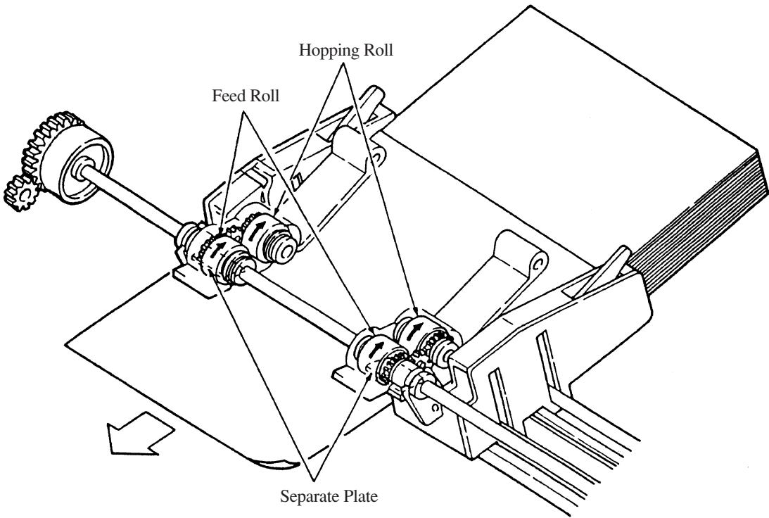
図 2-18. 自動給紙機構
