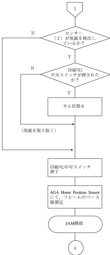
図 2-16. Jam 発生時フローチャート
