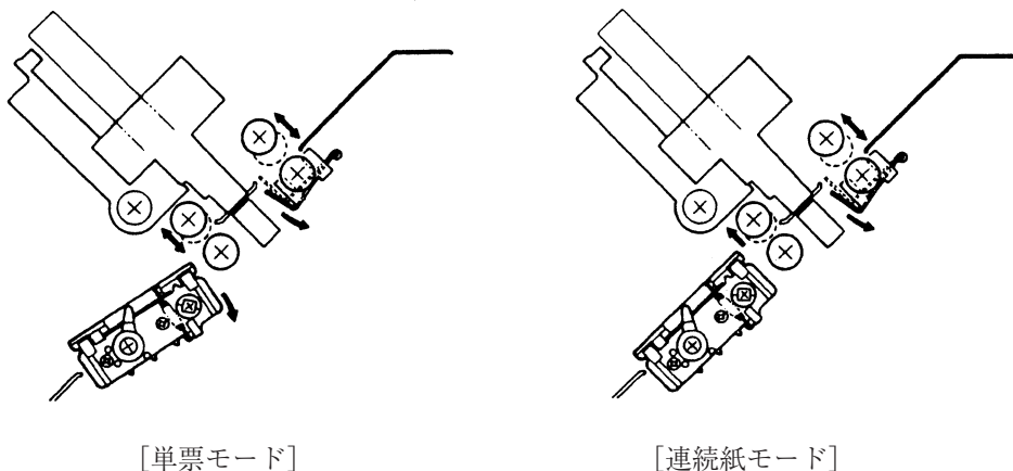
図 2-9. 連続用紙と単票用紙の走行系の状態
