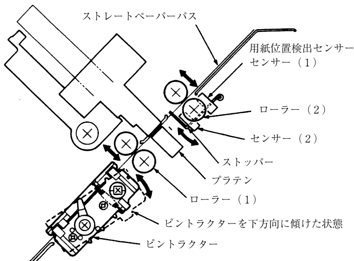
図 2-8. 用紙走行動作機構
