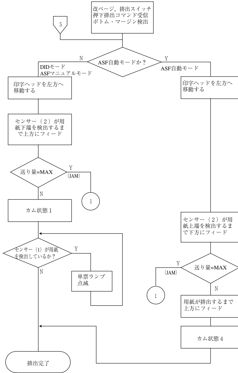
図 2-13. 単票排出フローチャート
