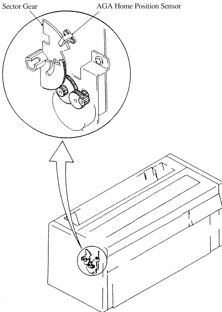
図 2-17. 自動用紙厚調整
