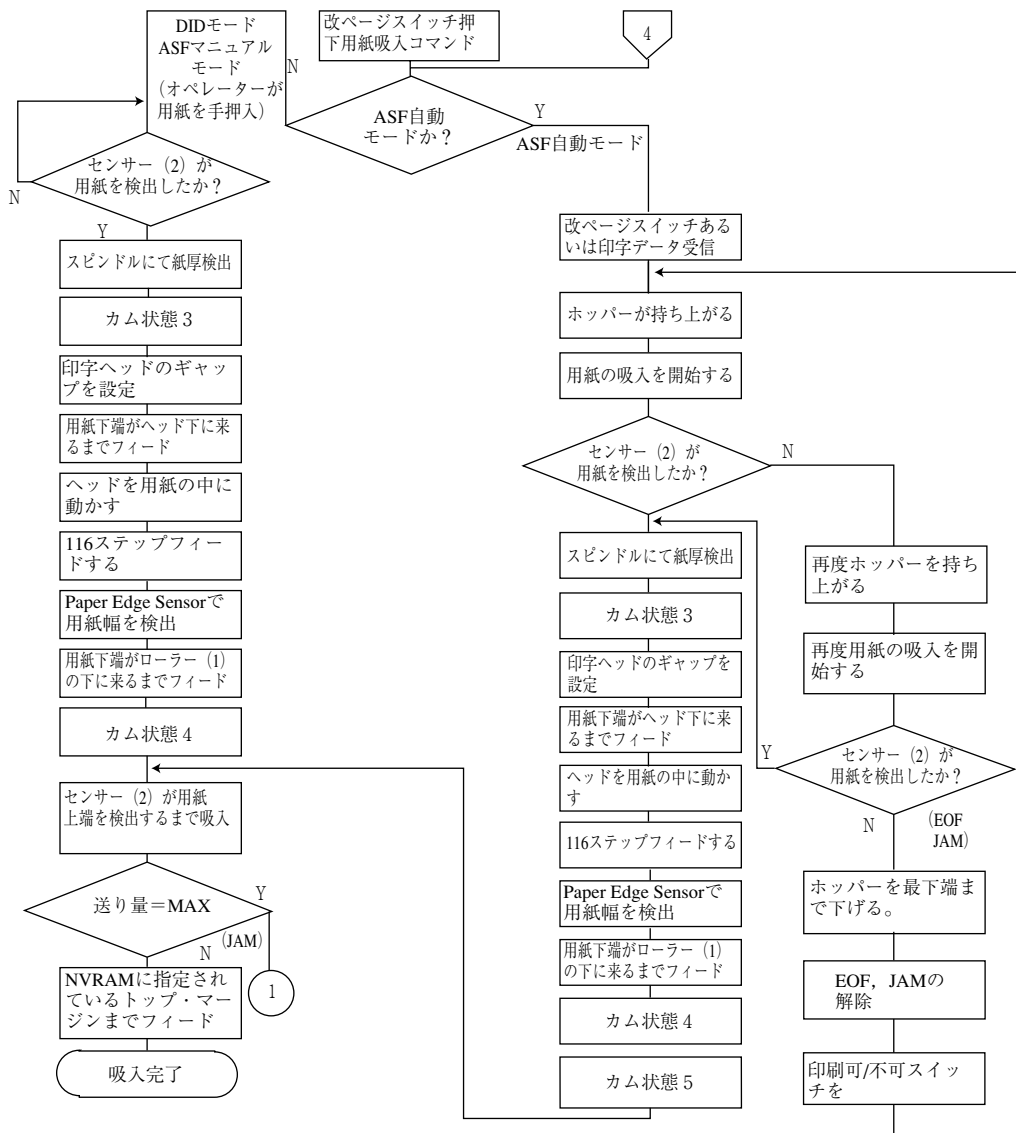
図 2-12. 単票吸入フローチャート
