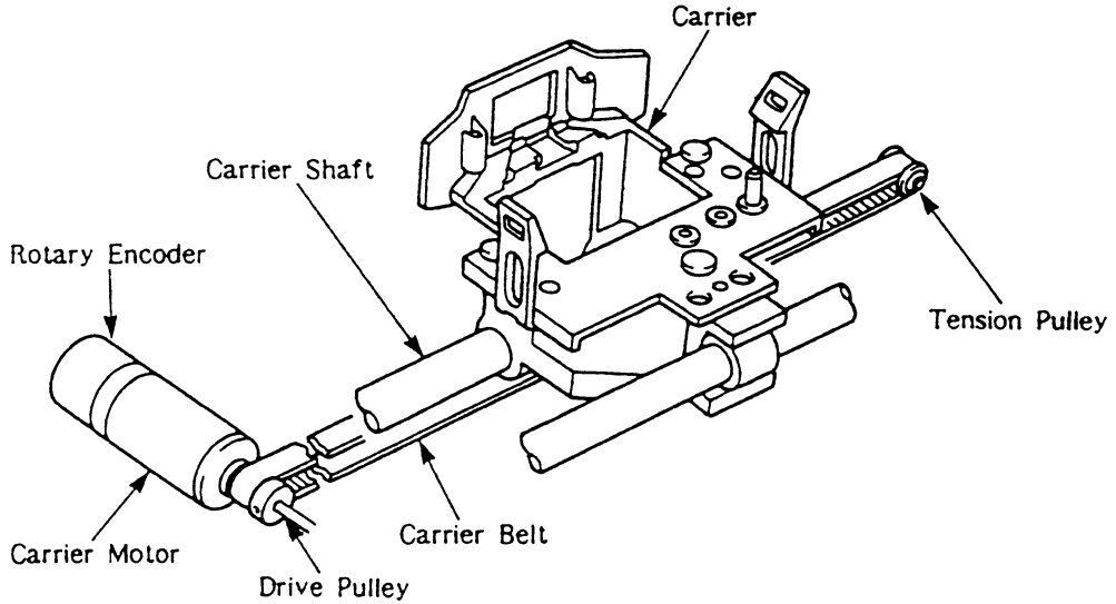
図 2-3. キャリアー・ドライブ機構
