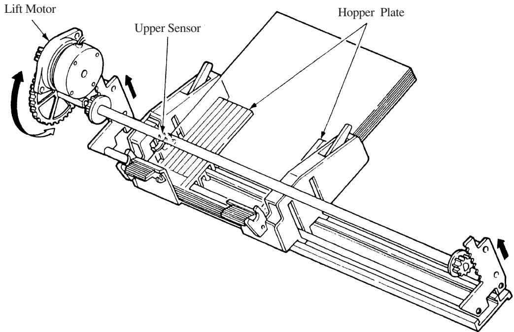
図 2-19. 自動給紙用紙リフト機構
