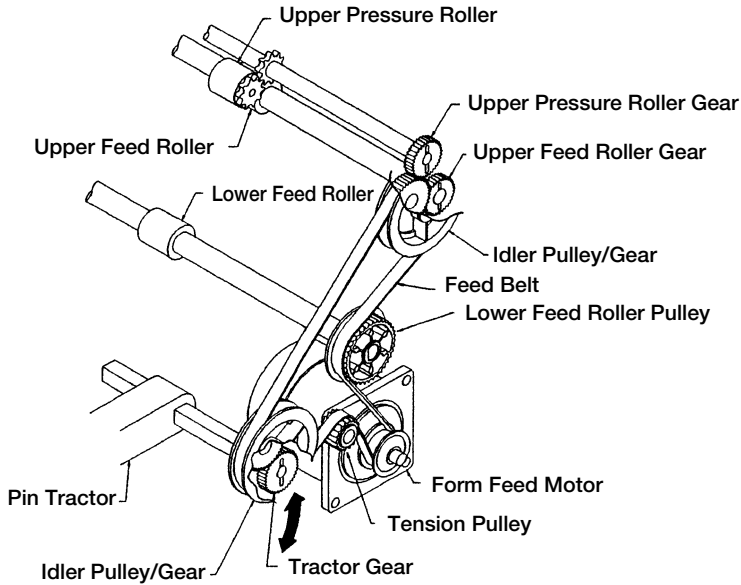
図 2-6. フォーム・フィード機構
