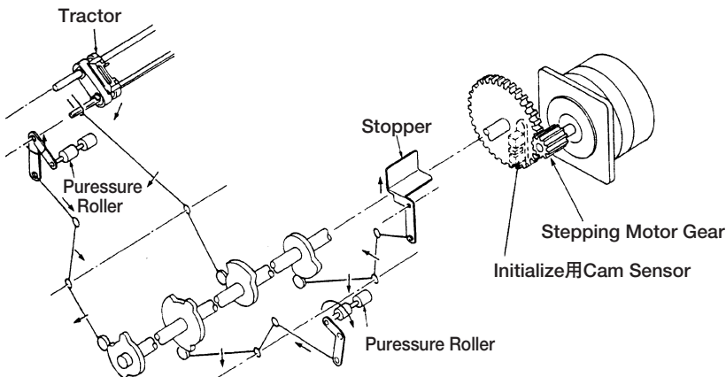
図 2-7. ローラー、トラクター、ストッパーのドライブ機構
