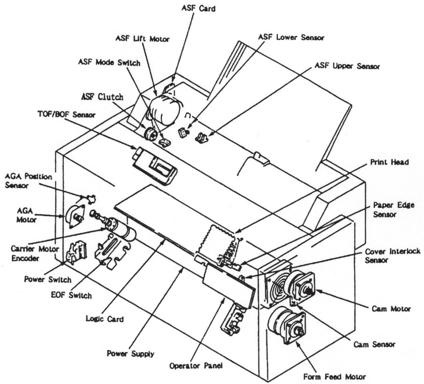
図4-2 電気部品配置図
