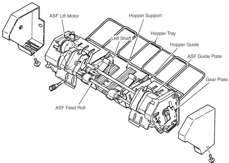
図4-3 ASFの主要部品配置図
