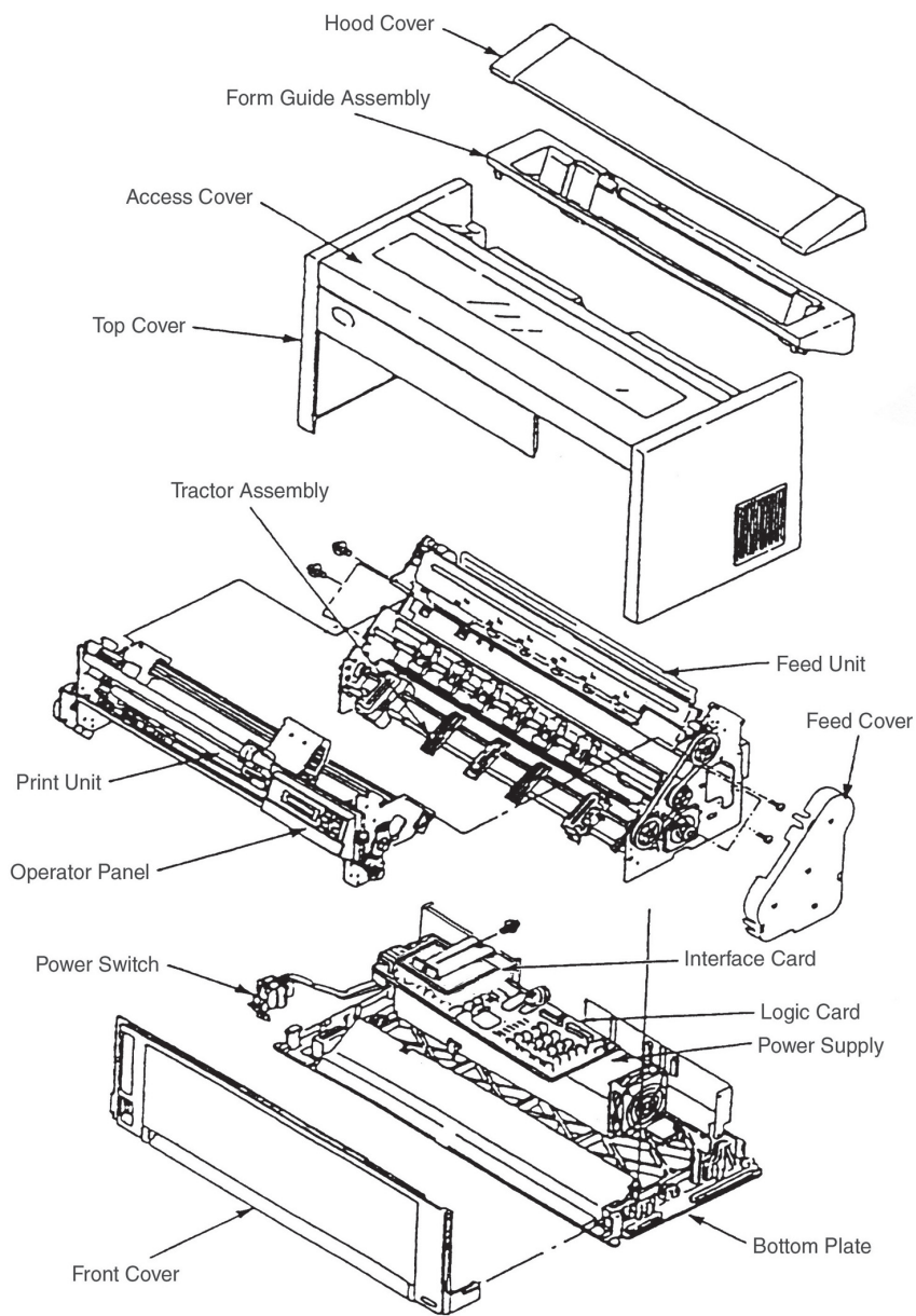
図4-1 InfoPrint 5577シリアル・プリンターの主要部品配置図
