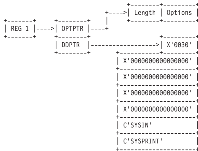
Figure 37. ICKDSF invocation parameter list
