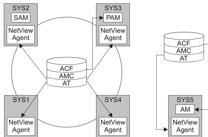
Figure 258. SA z/OS Automation Configuration
